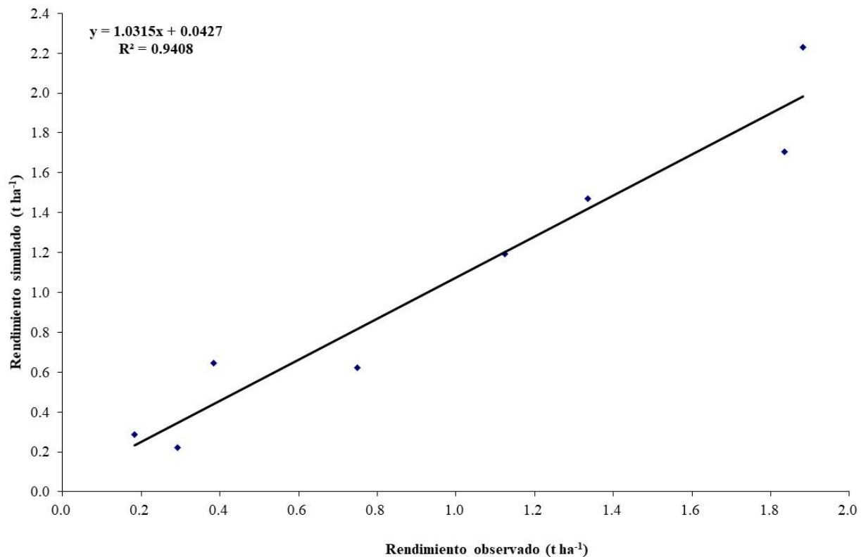
Figura 1.8. Coeficiente de determinación ( R^2 ) entre los valores de rendimiento de grano O i y S i con el modelo AquaCrop.
