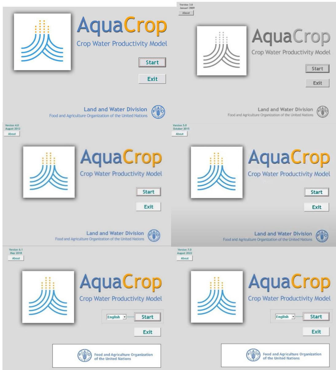
Figura 1. Evolución de las versiones del modelo AquaCrop a través del tiempo (2009-2022).
