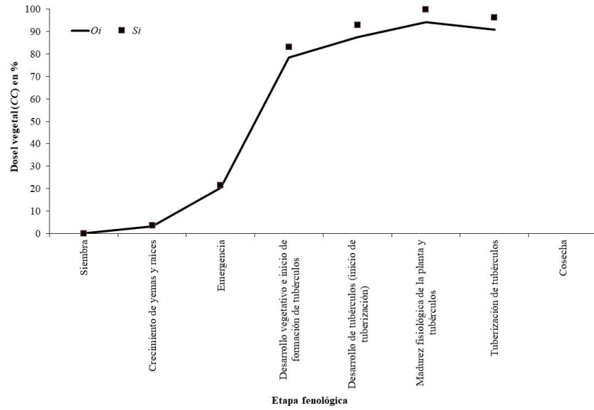
Figura 2.4. Comportamiento del dosel vegetal observado en campo ( Oi ) en comparación con la fenología simulada ( Si ) con AquaCrop en la variedad ‘Alpha’.
