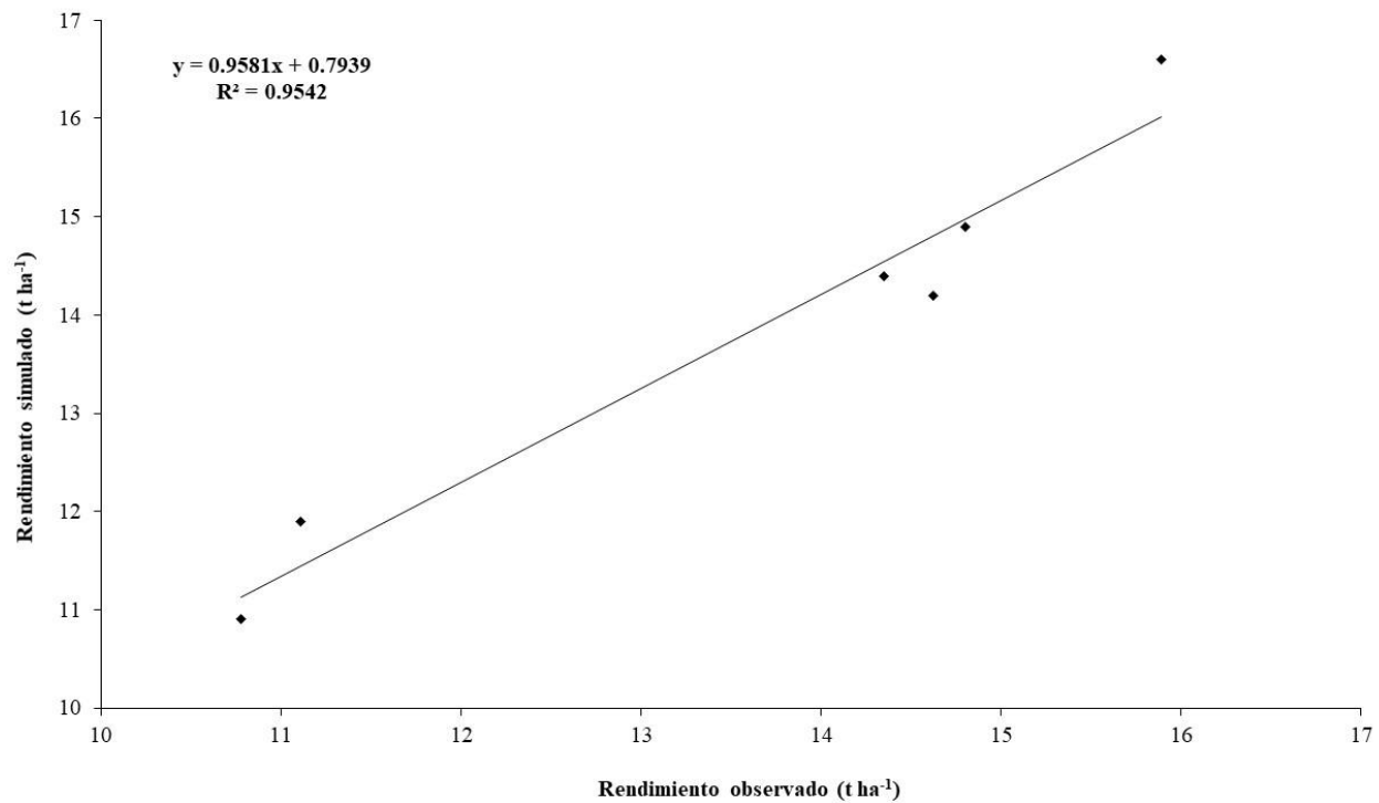
Figura 3.1. Coeficiente de determinación ( R^2 ) entre los valores de rendimiento de grano Oi y Si con el modelo AquaCrop.
