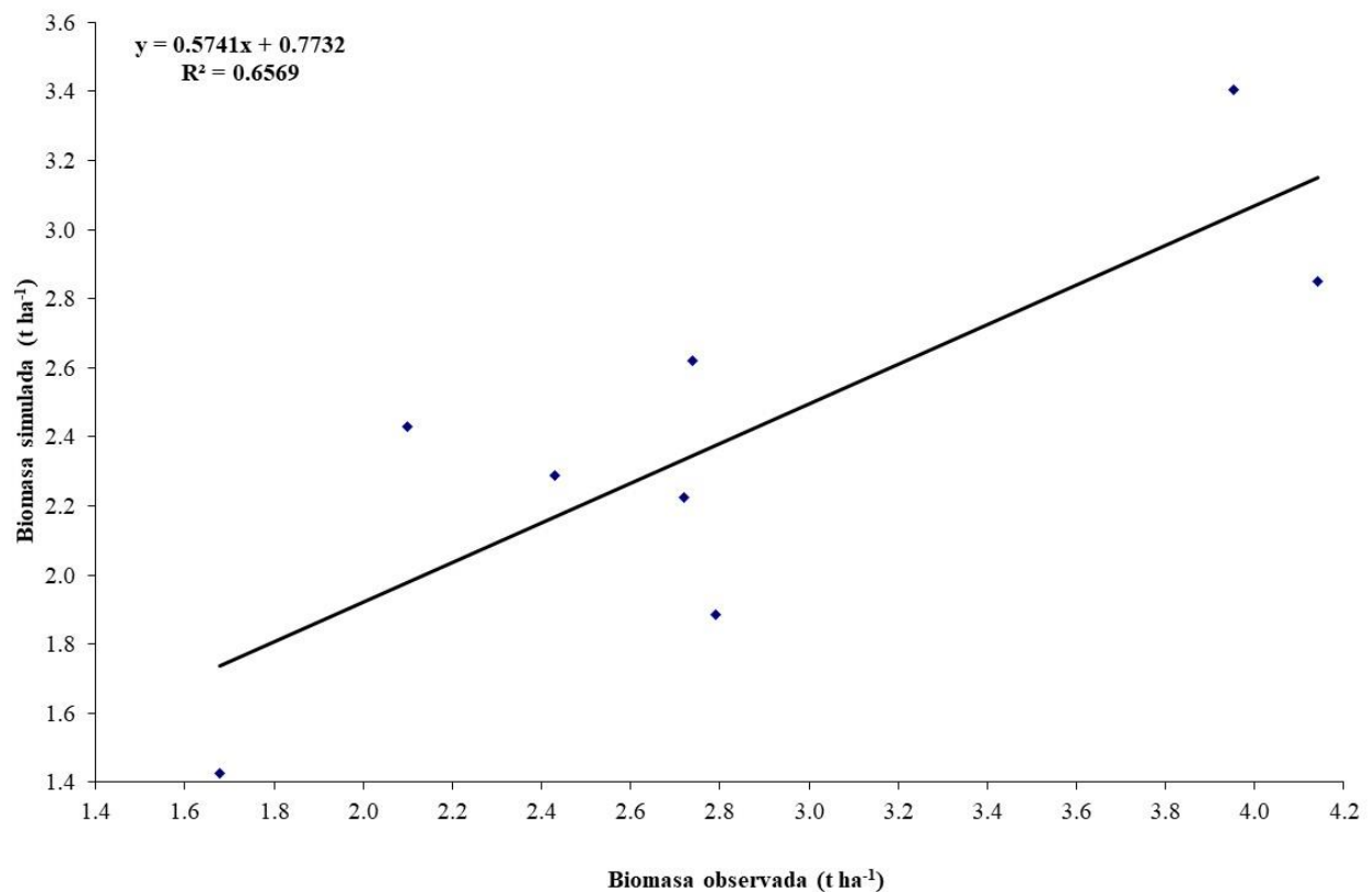
Figura 1.9. Coeficiente de determinación ( R^2 ) entre los valores de biomasa (B) Oi y Si con el modelo AquaCrop.
