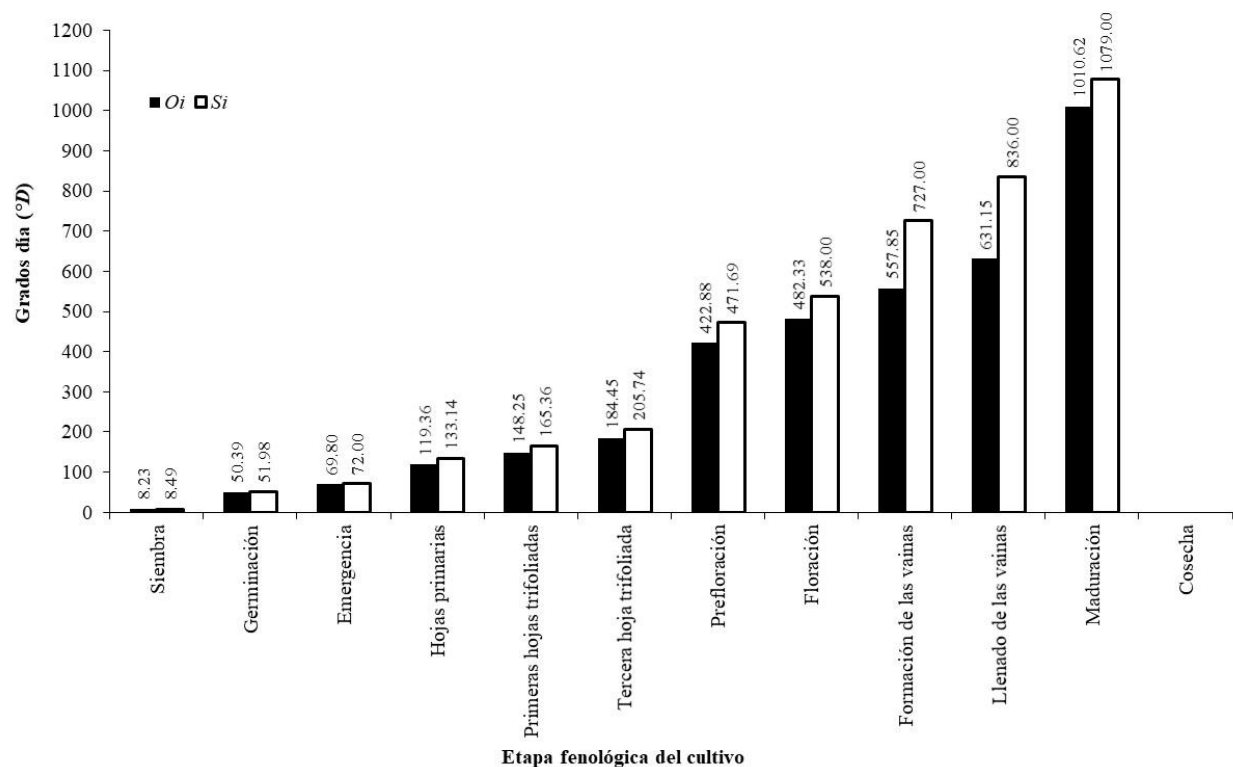
Figura 1.10. Comportamiento fenológico observado en campo (Oi) en comparación con la fenología simulada (Si) con AquaCrop.
