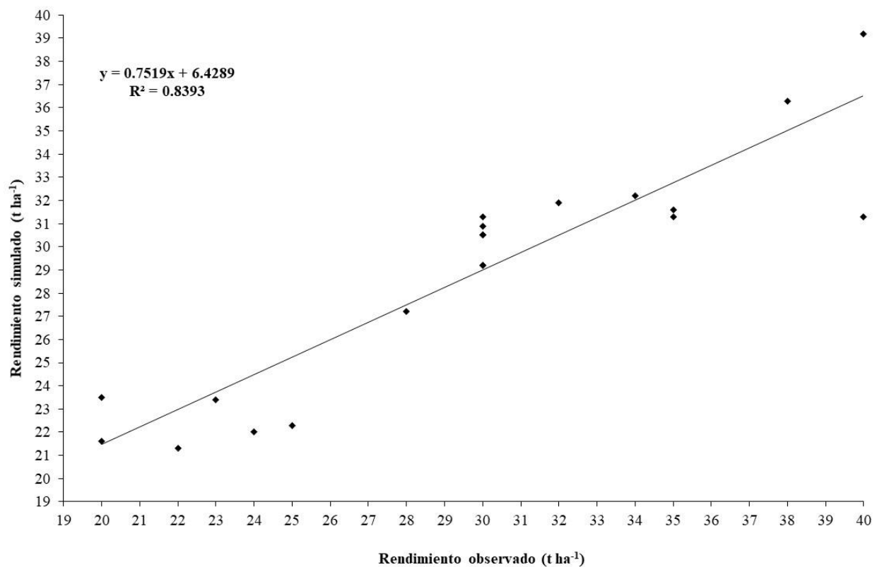
Figura 2.2. Coeficiente de determinación ( R^2 ) entre los valores de rendimiento de tubérculo Oi y Si con el modelo AquaCrop.
