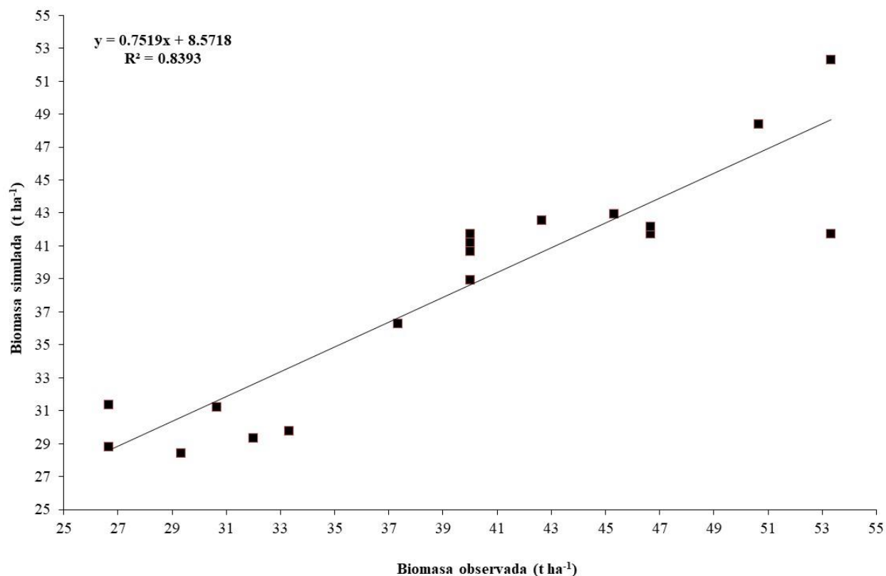
Figura 2.3. Coeficiente de determinación ( R^2 ) entre los valores de biomasa ( B ) O_i y S_i con el modelo AquaCrop.
