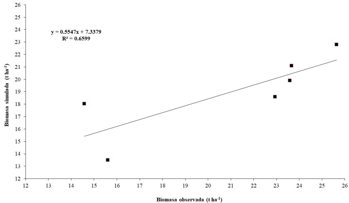
Figura 3.2. Coeficiente de determinación ( R^2 ) entre los valores de B\ O_i y B\ S_i con el modelo AquaCrop.
