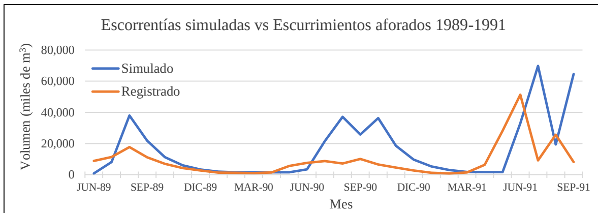
Figura 4.34.- Resultados de escorrentías simuladas contra escurrimientos aforados para la segunda evaluación del código.
