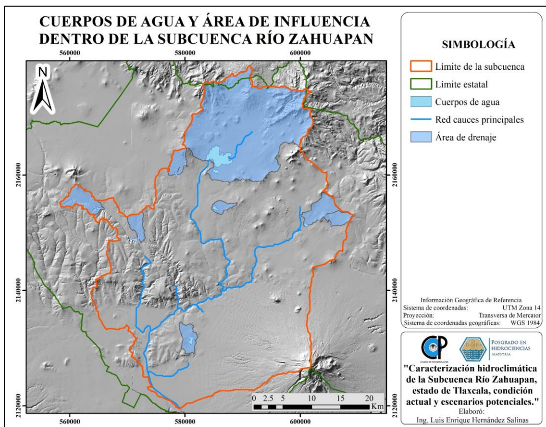
Figura 4.7.- Áreas de drenaje de los cuerpos de agua dentro de la subcuenca río Zahuapan.
