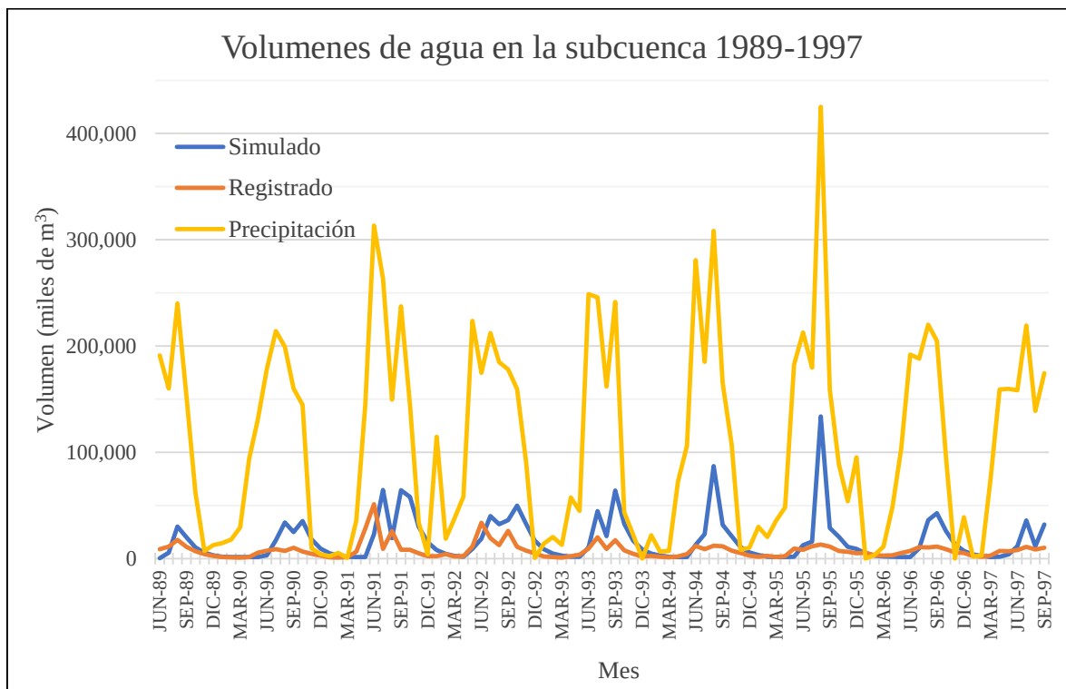
Figura 4.35.- Comportamiento de las escorrentías simuladas y escurrimientos aforados en respuesta a la precipitación total en la subcuenca.
