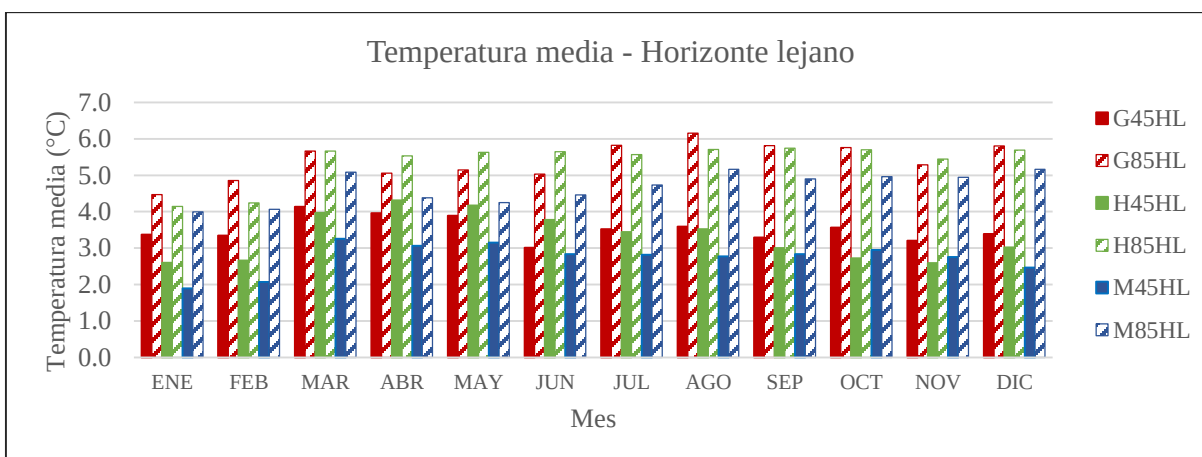
Figura 5.23.- Diferencia de la temperatura media mensual promedio en la subcuenca para los escenarios en el horizonte lejano (2075-2099).
