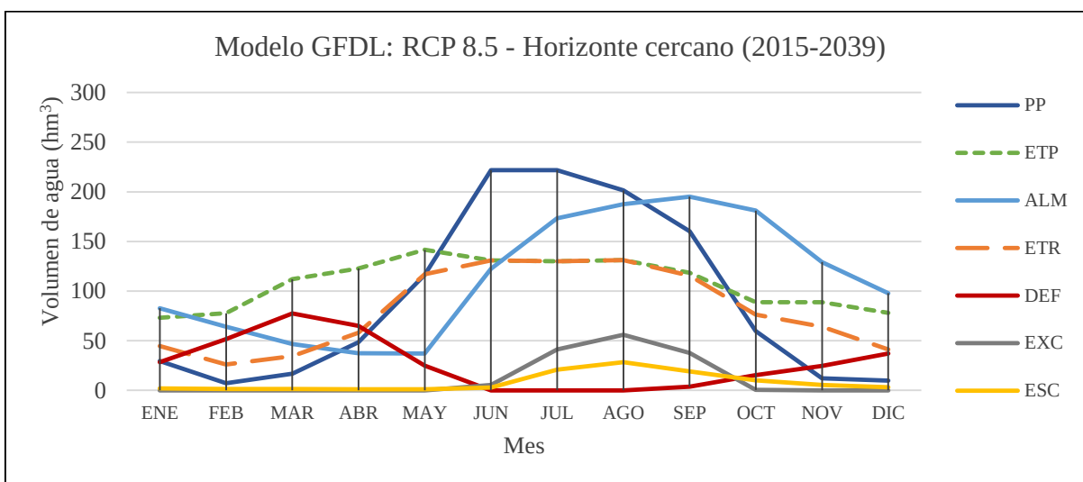
Figura 5.12.- Comportamiento del balance hídrico de la subcuenca río Zahuapan bajo el escenario RCP8.5 en el horizonte cercano (2015-2039) respectivo al modelo GFDL.
