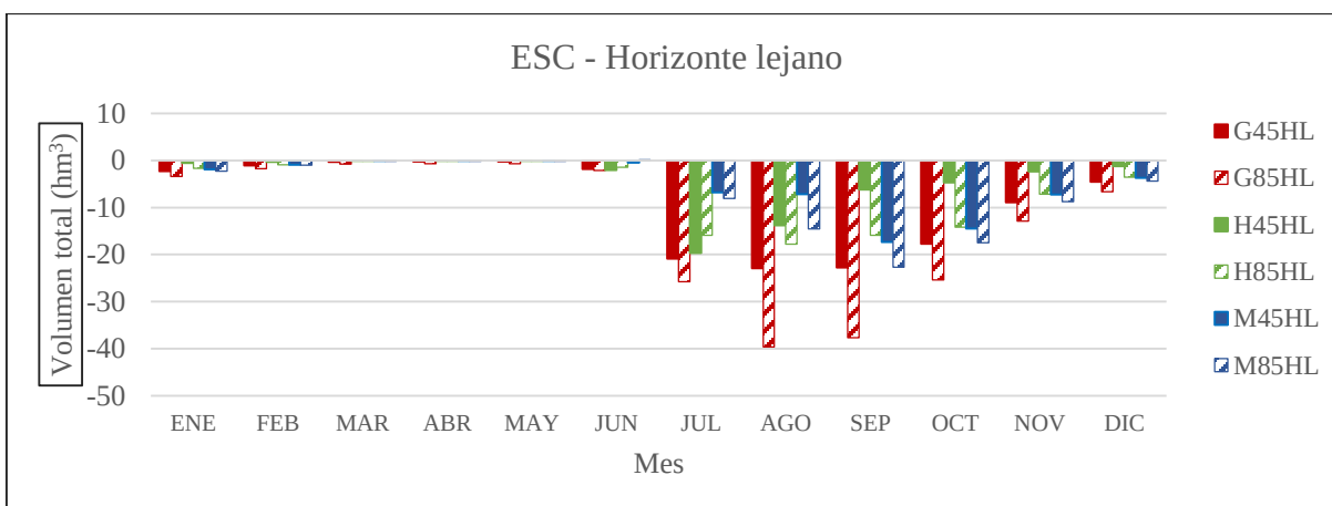
Figura 5.35.- Diferencia del volumen de escorrentía total en la subcuenca para los escenarios en el horizonte lejano (2075-2099) con respecto a la línea base.
