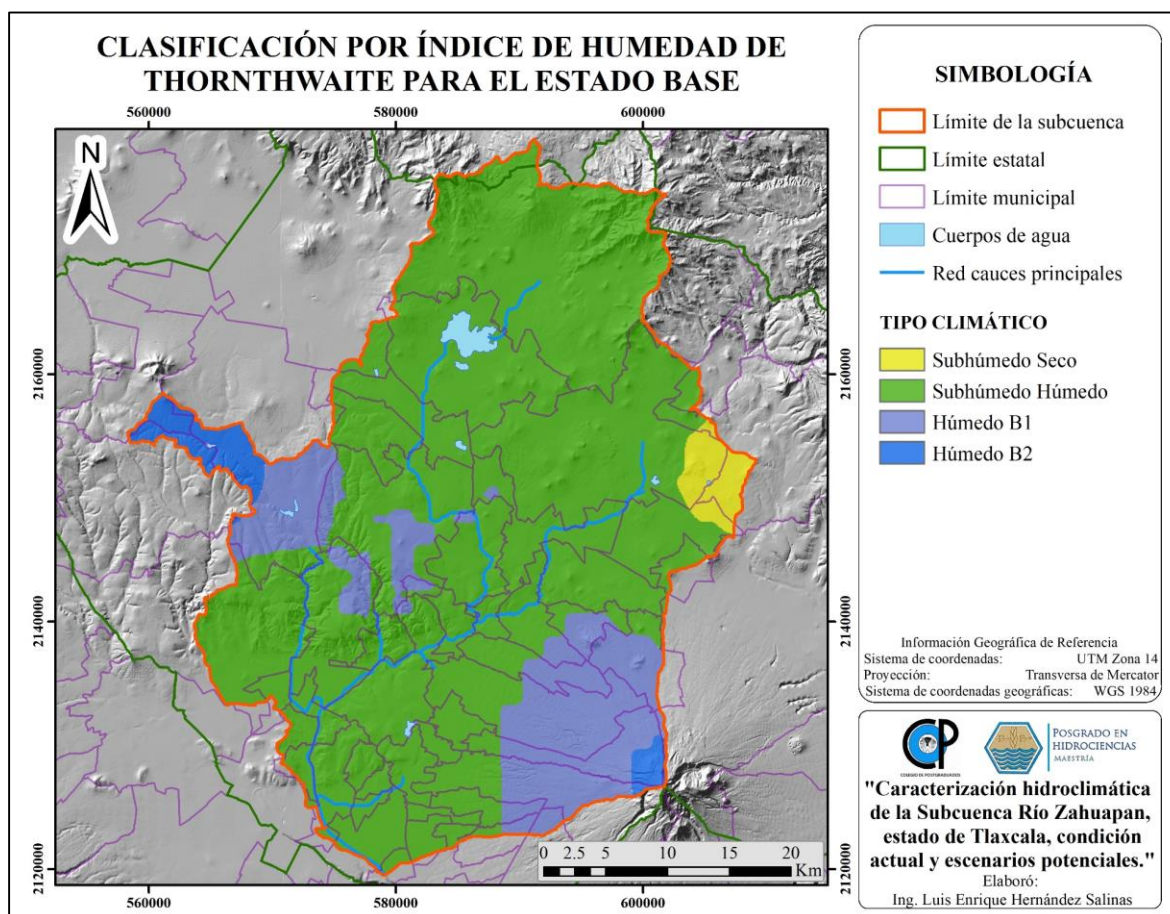
Figura 5.3.- Distribución de climas por índice de humedad para el estado base.
