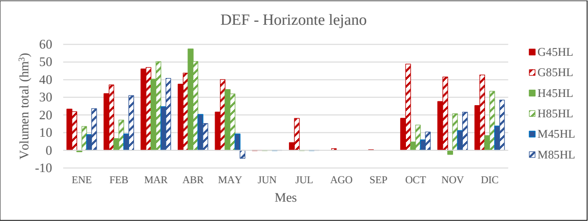
Figura 5.31.- Diferencia del volumen de déficit de agua total en la subcuenca para los escenarios en el horizonte lejano (2075-2099) con respecto a la línea base.
