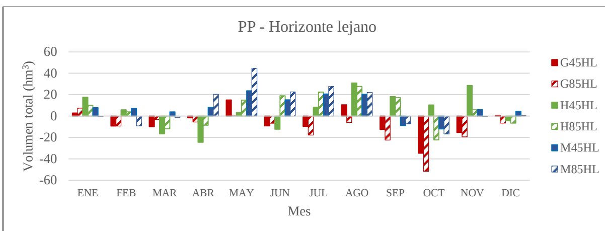
Figura 5.21.- Diferencia del volumen de precipitación total en la subcuenca para los escenarios en el horizonte lejano (2075-2099) con respecto a la línea base.
