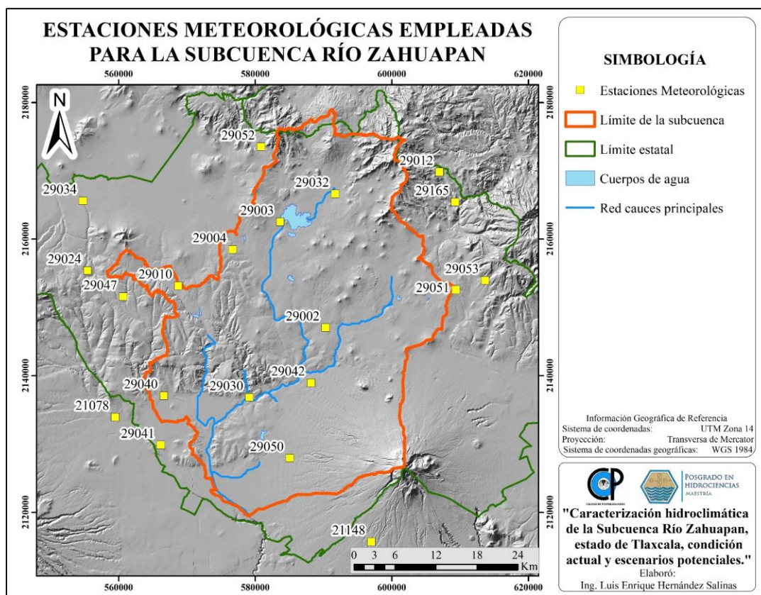
Figura 4.22.- Distribución espacial de las estaciones meteorológicas seleccionadas.
