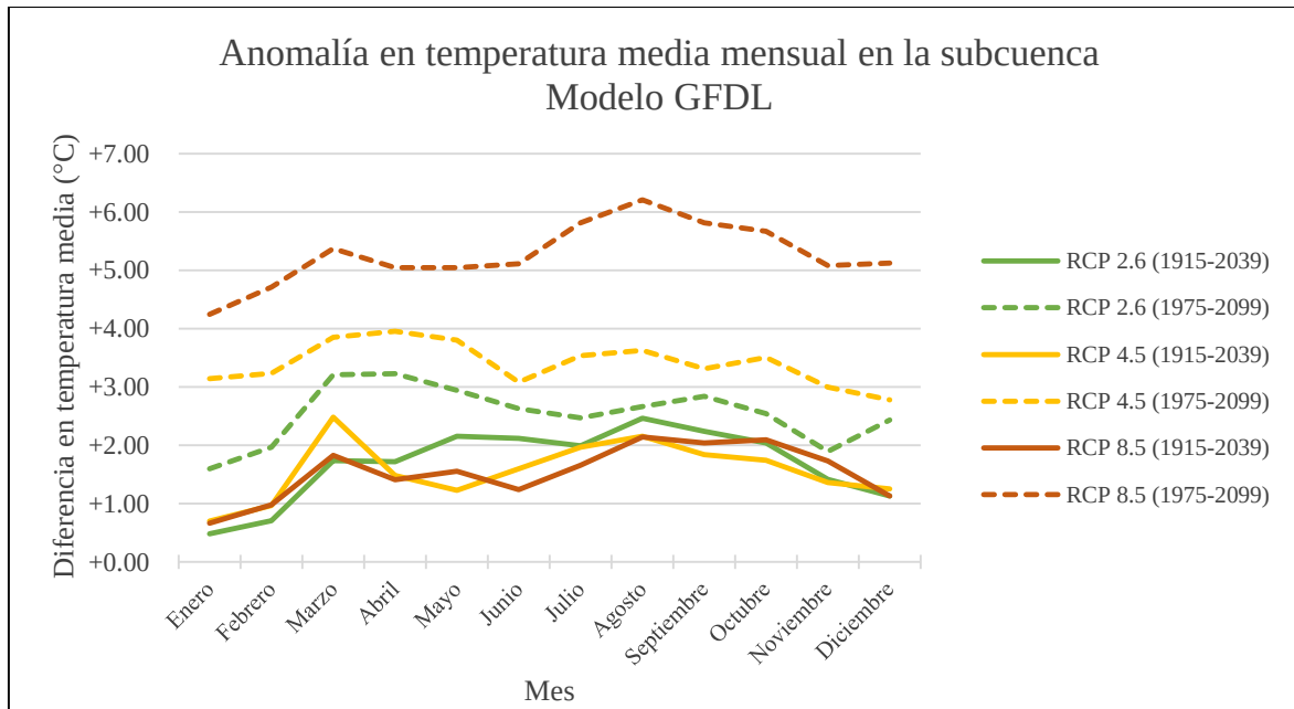
Figura 4.24.- Anomalía esperada en Temperatura media mensual bajo MCG GFDL_CM3 en la subcuenca.
