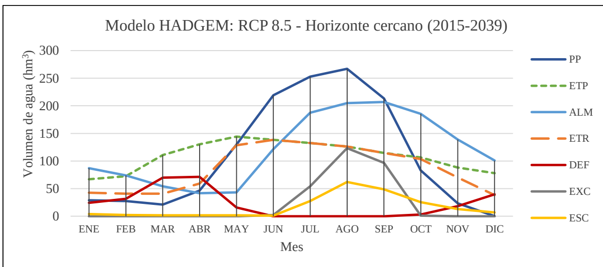
Figura 5.13.- Comportamiento del balance hídrico de la subcuenca río Zahuapan bajo el escenario RCP8.5 en el horizonte cercano (2015-2039) respectivo al modelo HADGEM.
