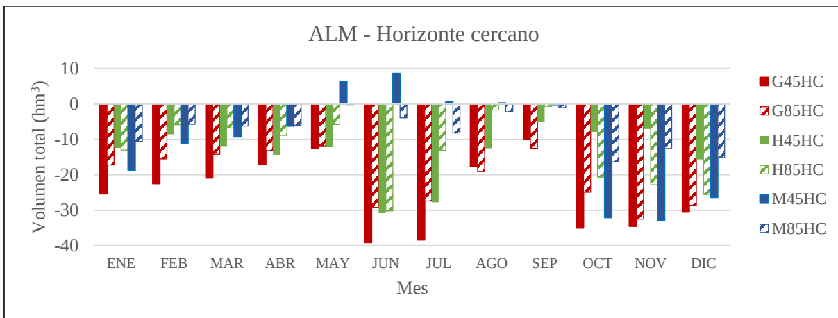
Figura 5.28.- Diferencia del volumen de agua almacenada en el suelo total en la subcuenca para los escenarios en el horizonte cercano (2015-2039) con respecto a la línea base.
