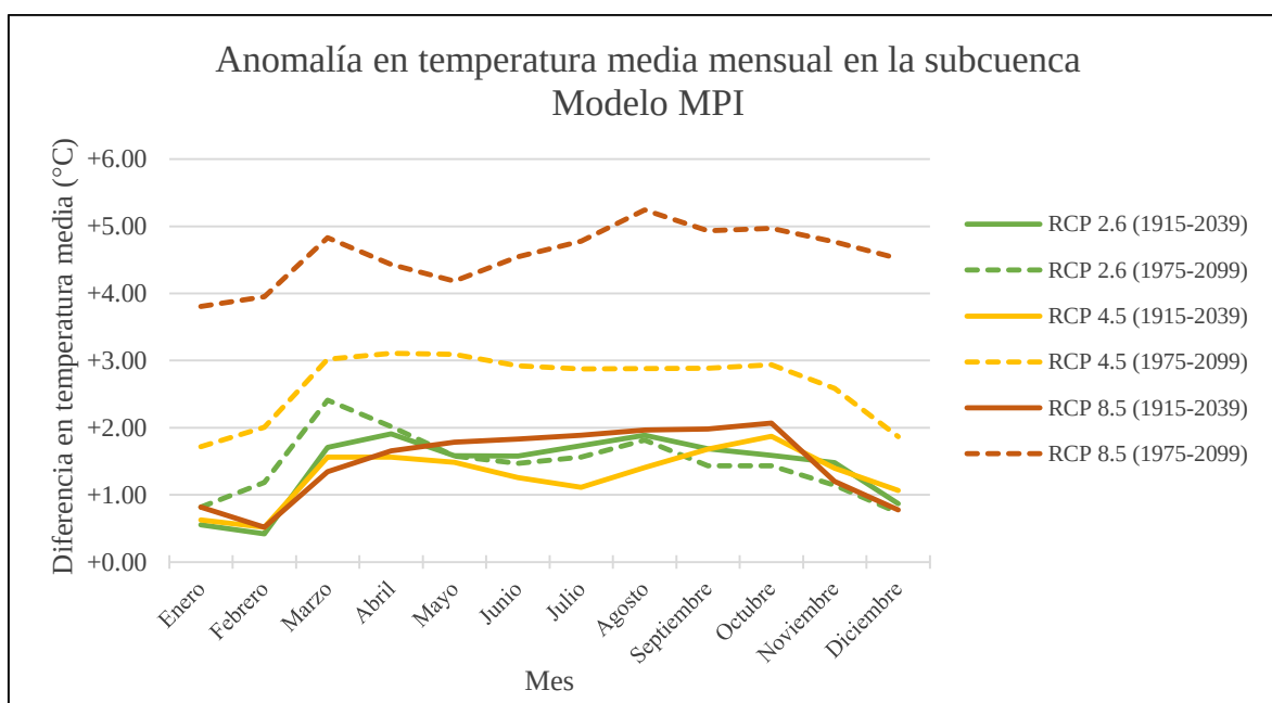
Figura 4.28.- Anomalía esperada en Temperatura media mensual bajo MCG MPI_ESM_LR en la subcuenca.
