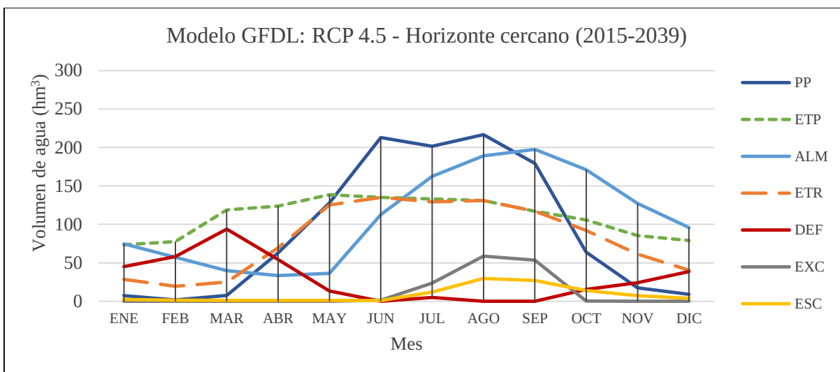
Figura 5.4.- Comportamiento del balance hídrico de la subcuenca río Zahuapan bajo el escenario RCP4.5 en el horizonte cercano (2015-2039) respectivo al modelo GFDL.
