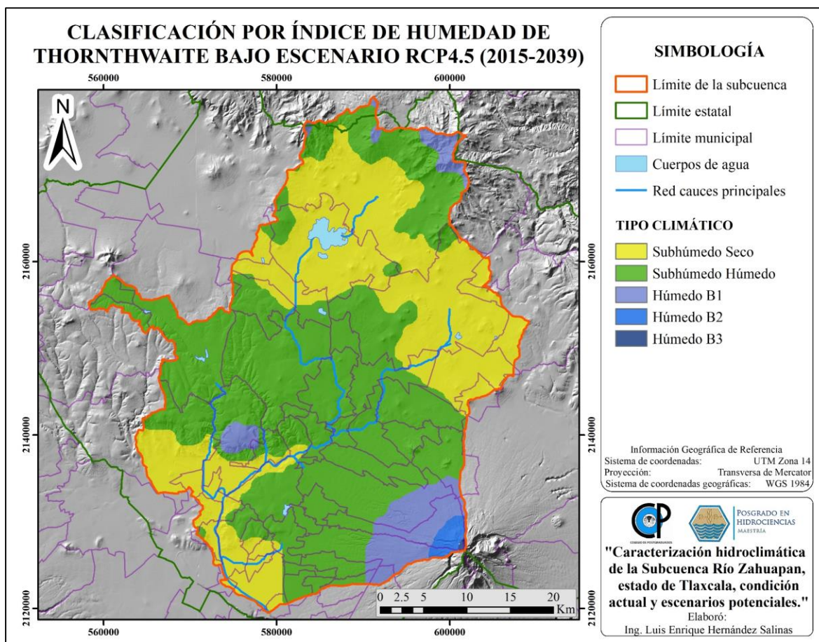
Figura 5.7.- Distribución de climas por índice de humedad para el escenario RCP4.5 (2015-2039).
