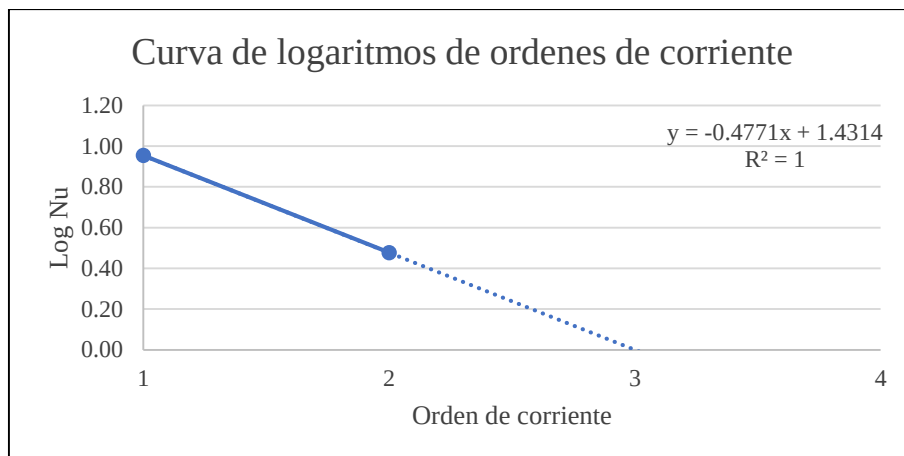
Figura 4.20.- Curva de logaritmos de relaciones de bifurcación.
