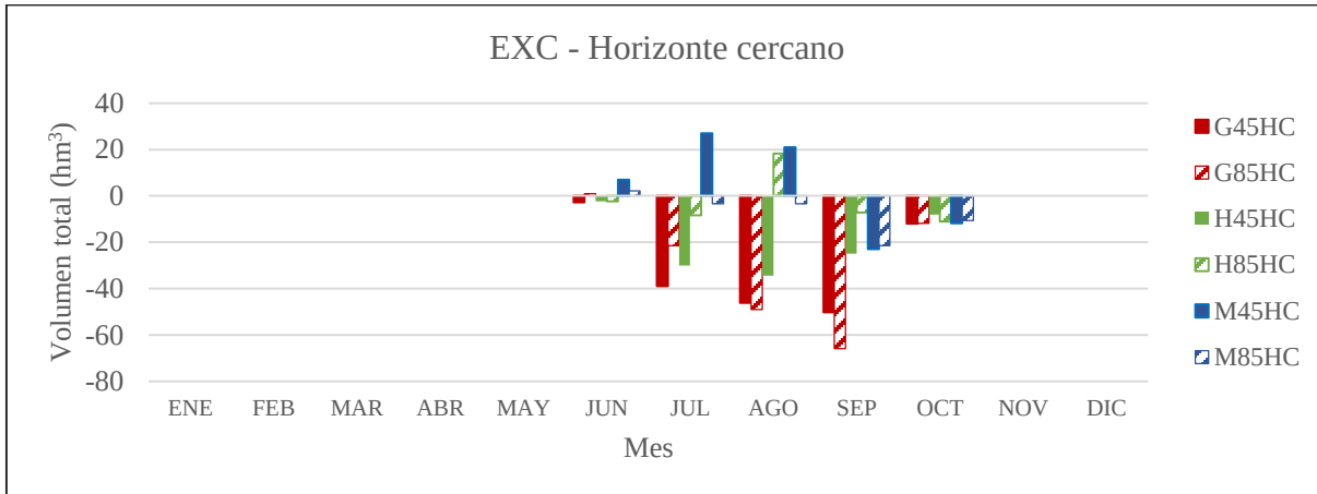
Figura 5.32.- Diferencia del volumen de exceso de humedad total en la subcuenca para los escenarios en el horizonte cercano (2015-2039) con respecto a la línea base.
