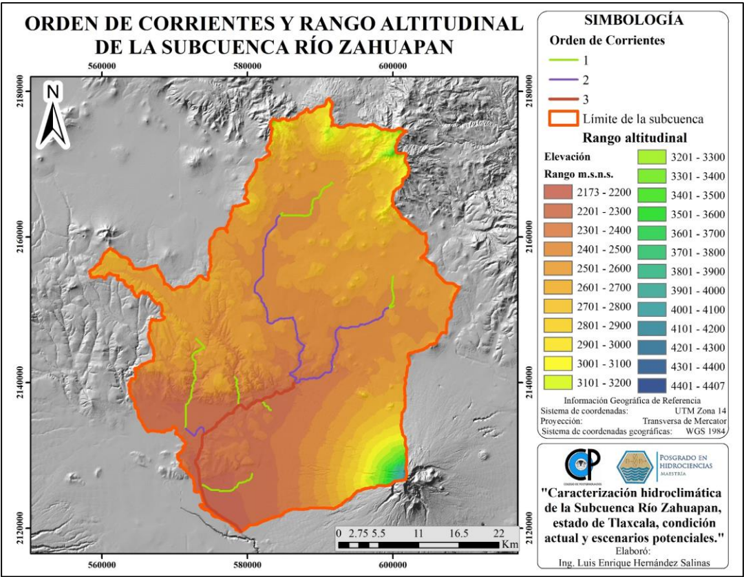
Figura 4.19.- Ordenes de corrientes presentes en la cuenca.
