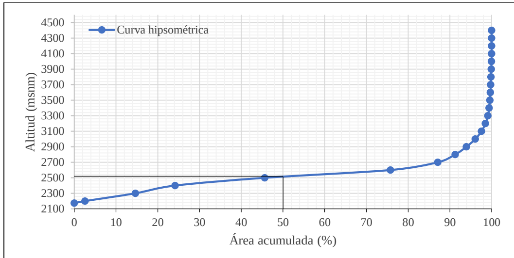
Figura 4.21.- Curva hipsométrica desarrollada para la cuenca.
