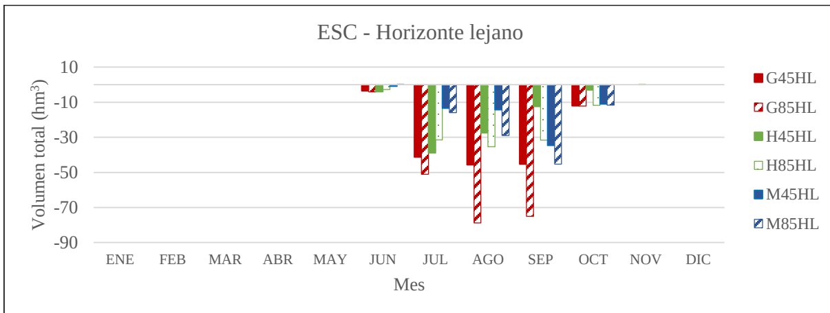
Figura 5.33.- Diferencia del volumen de exceso de humedad total en la subcuenca para los escenarios en el horizonte lejano (2075-2099) con respecto a la línea base.
