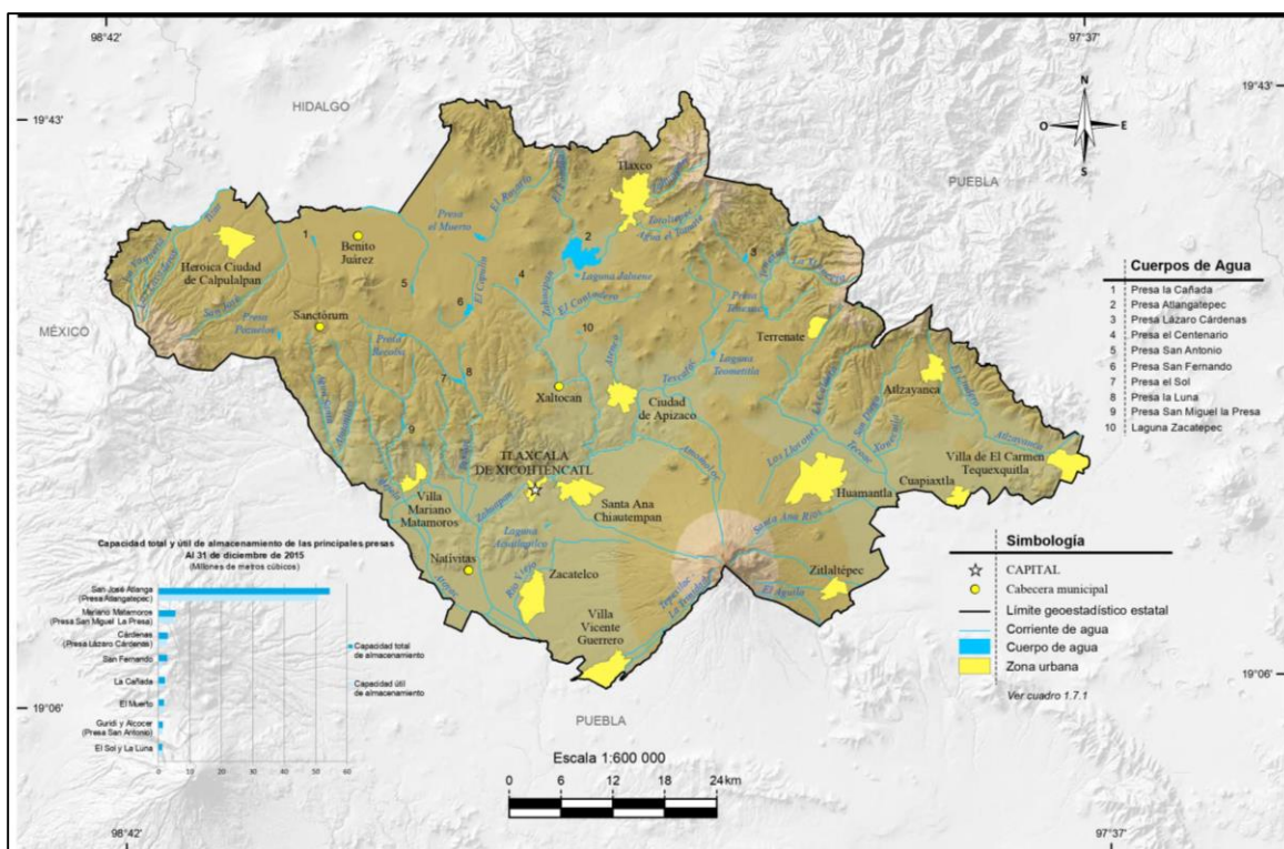
Figura 4.6.- Principales cauces y cuerpos de agua en el estado de Tlaxcala.
