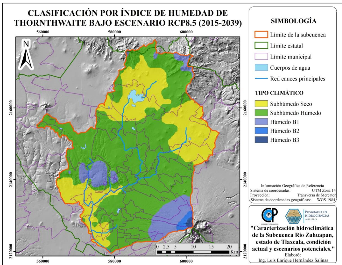
Figura 5.15.- Distribución de climas por índice de humedad para el escenario RCP8.5 (2015-2039).
