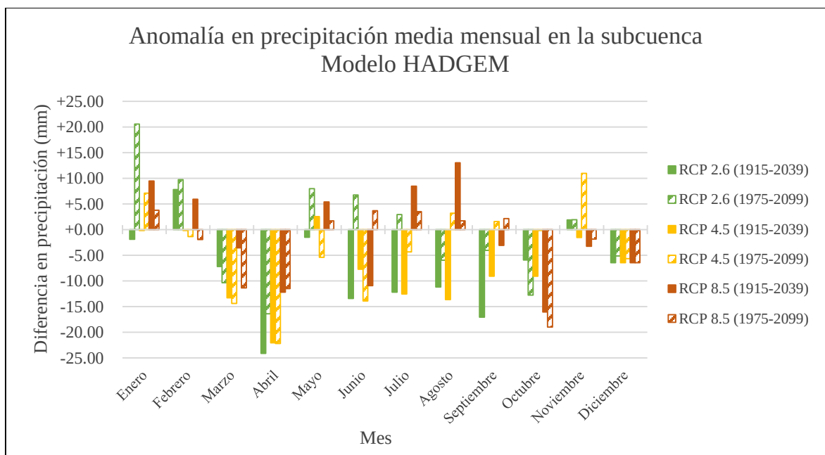
Figura 4.25.- Anomalía esperada en PP media mensual bajo MCG HADGEM2_ES en la subcuenca.
