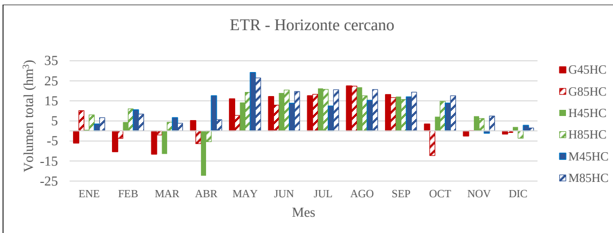
Figura 5.26.- Diferencia del volumen de evapotranspiración real total en la subcuenca para los escenarios en el horizonte cercano (2015-2039) con respecto a la línea base.
