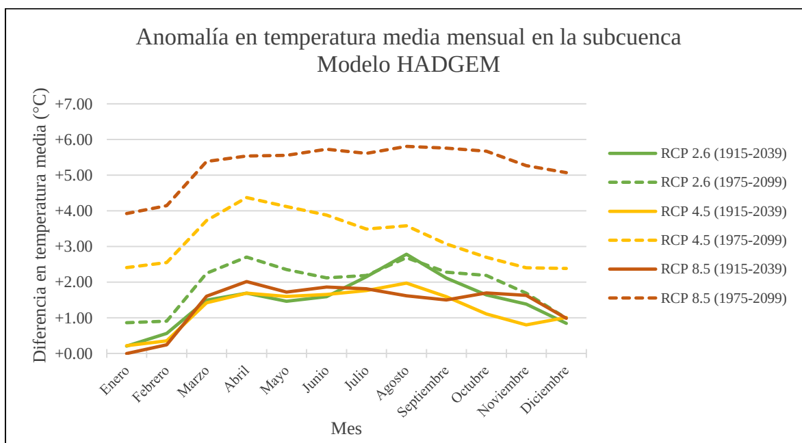
Figura 4.26.- Anomalía esperada en Temperatura media mensual bajo MCG HADGEM2_ES en la subcuenca.
