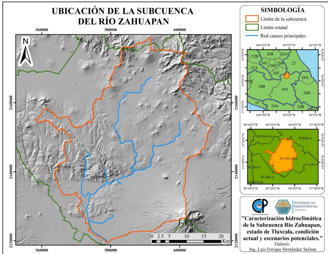
Figura 4.1.- Ubicación y aspecto de la subcuenca del río Zahuapan, Tlaxcala.
