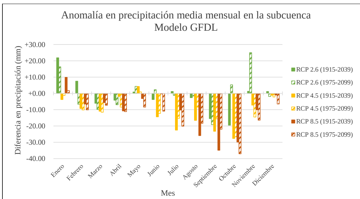
Figura 4.23.- Anomalía esperada en PP media mensual bajo MCG GFDL_CM3 en la subcuenca.
