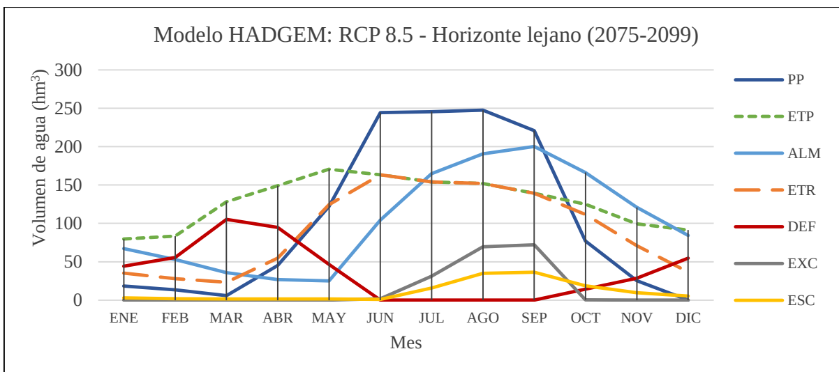
Figura 5.17.- Comportamiento del balance hídrico de la subcuenca río Zahuapan bajo el escenario RCP8.5 en el horizonte lejano (2075-2099) respectivo al modelo HADGEM.
