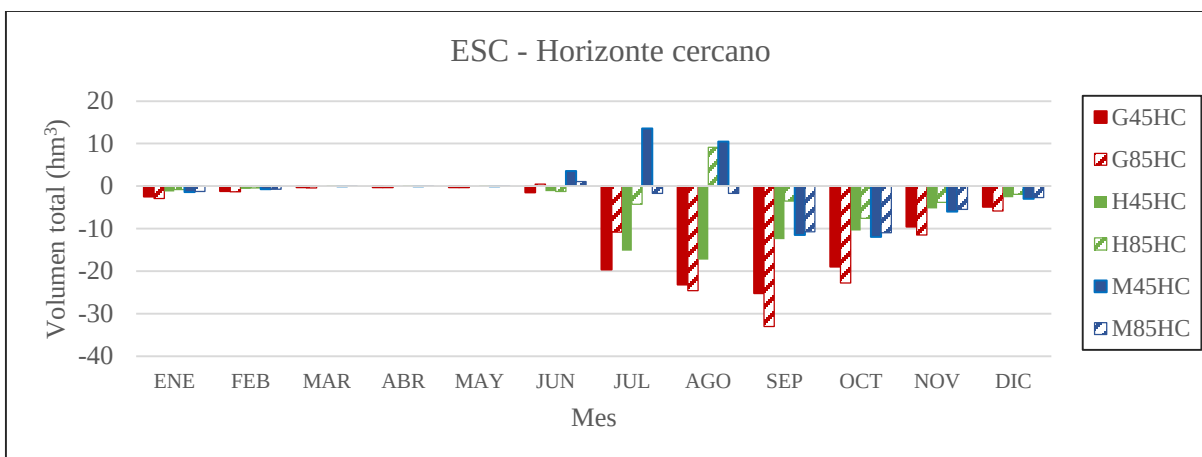
Figura 5.34.- Diferencia del volumen de escorrentía total en la subcuenca para los escenarios en el horizonte cercano (2015-2039) con respecto a la línea base.
