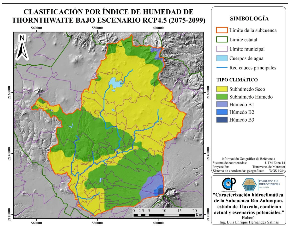
Figura 5.11.- Distribución de climas por índice de humedad para el escenario RCP4.5 (2075-2099).
