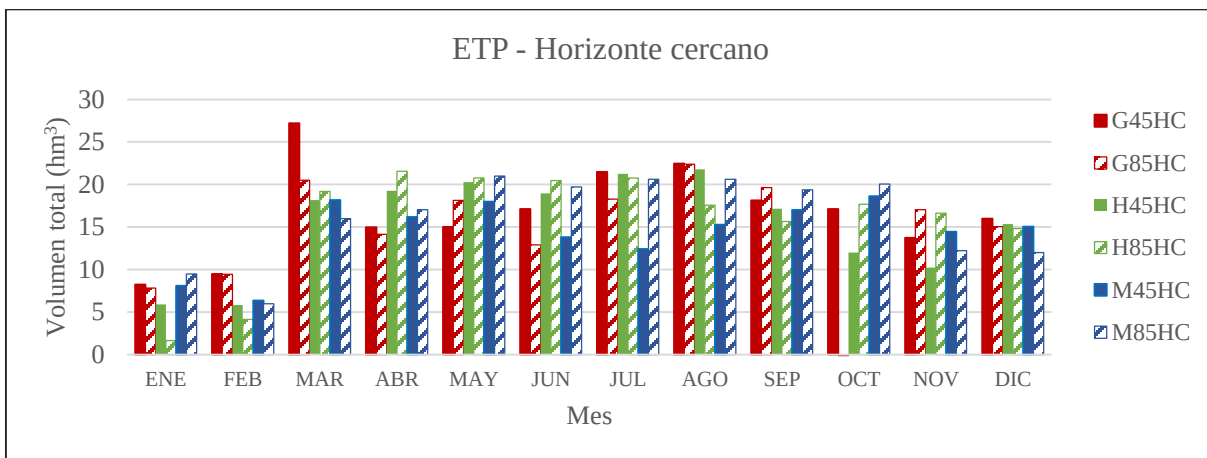
Figura 5.24.- Diferencia del volumen de evapotranspiración potencial total en la subcuenca para los escenarios en el horizonte cercano (2015-2039) con respecto a la línea base.
