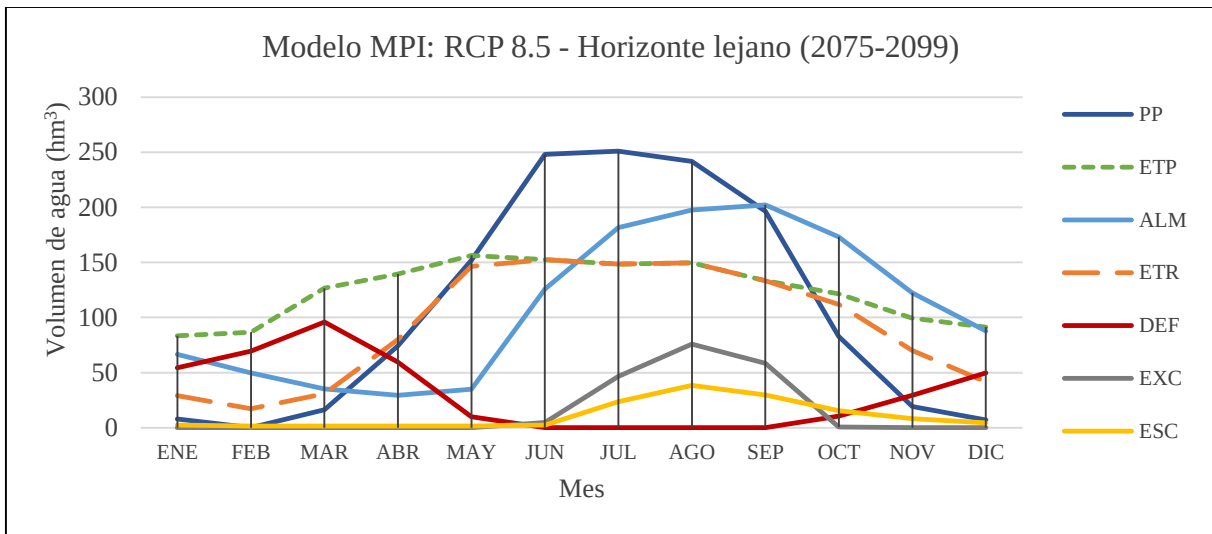
Figura 5.18.- Comportamiento del balance hídrico de la subcuenca río Zahuapan bajo el escenario RCP8.5 en el horizonte lejano (2075-2099) respectivo al modelo MPI.
