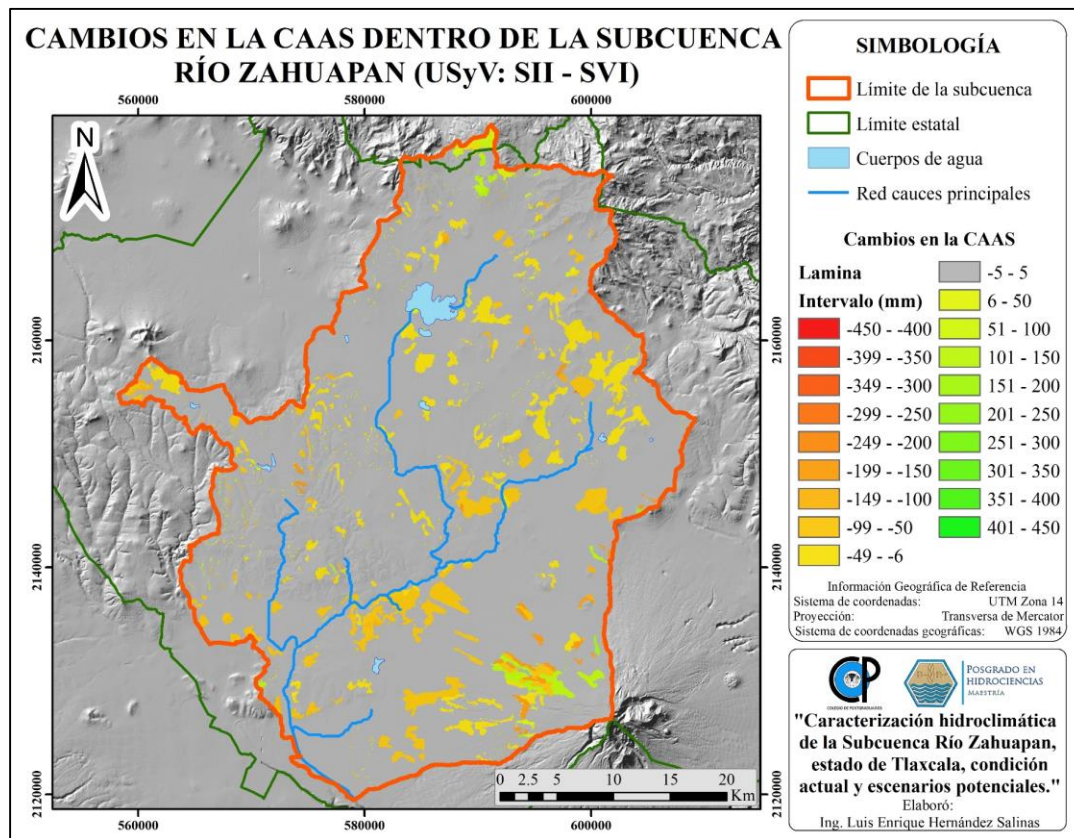
Figura 5.1.- Modificaciones en la Capacidad de almacenamiento de agua en el suelo entre las Series II y VI de INEGI.
