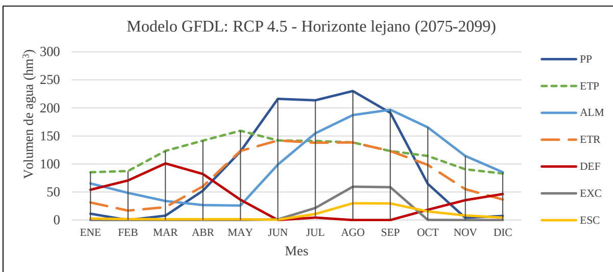
Figura 5.8.- Comportamiento del balance hídrico de la subcuenca río Zahuapan bajo el escenario RCP4.5 en el horizonte lejano (2075-2099) respectivo al modelo GFDL.
