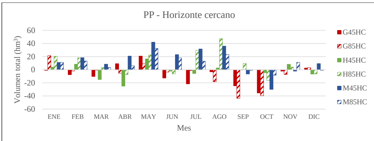
Figura 5.20.- Diferencia del volumen de precipitación total en la subcuenca para los escenarios en el horizonte cercano (2015-2039) con respecto a la línea base.
