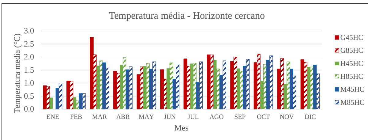
Figura 5.22.- Diferencia de la temperatura media mensual promedio en la subcuenca para los escenarios en el horizonte cercano (2015-2039) con respecto a la línea base.
