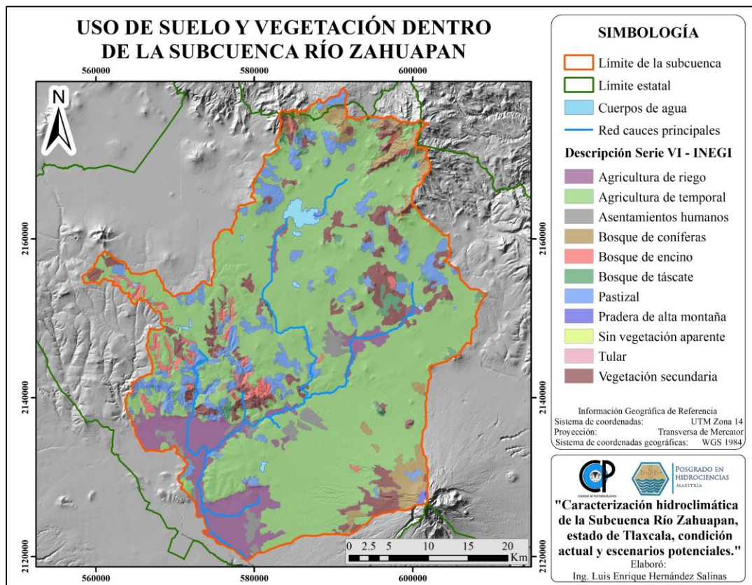
Figura 4.8.- Uso de Suelo y Vegetación en la subcuenca del río Zahuapan.
