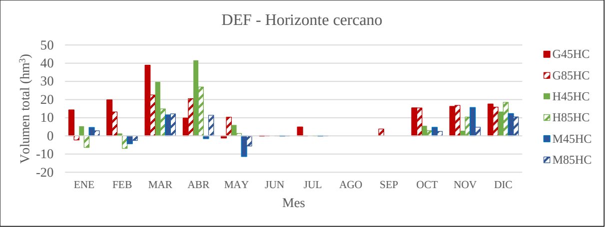
Figura 5.30.- Diferencia del volumen de déficit de agua total en la subcuenca para los escenarios en el horizonte cercano (2015-2039) con respecto a la línea base.
