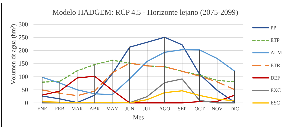
Figura 5.9.- Comportamiento del balance hídrico de la subcuenca río Zahuapan bajo el escenario RCP4.5 en el horizonte lejano (2075-2099) respectivo al modelo HADGEM.
