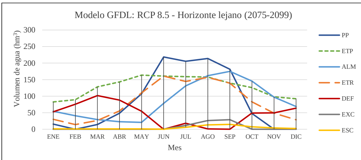
Figura 5.16.- Comportamiento del balance hídrico de la subcuenca río Zahuapan bajo el escenario RCP8.5 en el horizonte lejano (2075-2099) respectivo al modelo GFDL.
