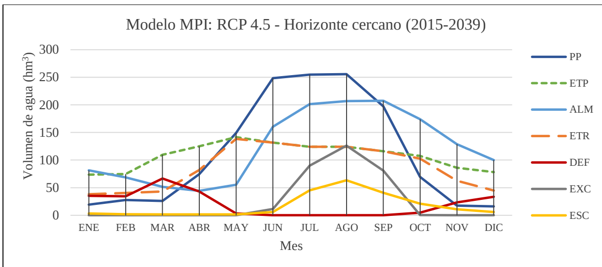
Figura 5.6.- Comportamiento del balance hídrico de la subcuenca río Zahuapan bajo el escenario RCP4.5 en el horizonte cercano (2015-2039) respectivo al modelo MPI.
