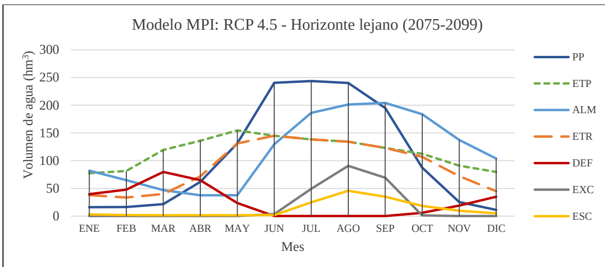
Figura 5.10.- Comportamiento del balance hídrico de la subcuenca río Zahuapan bajo el escenario RCP4.5 en el horizonte lejano (2075-2099) respectivo al modelo MPI.
