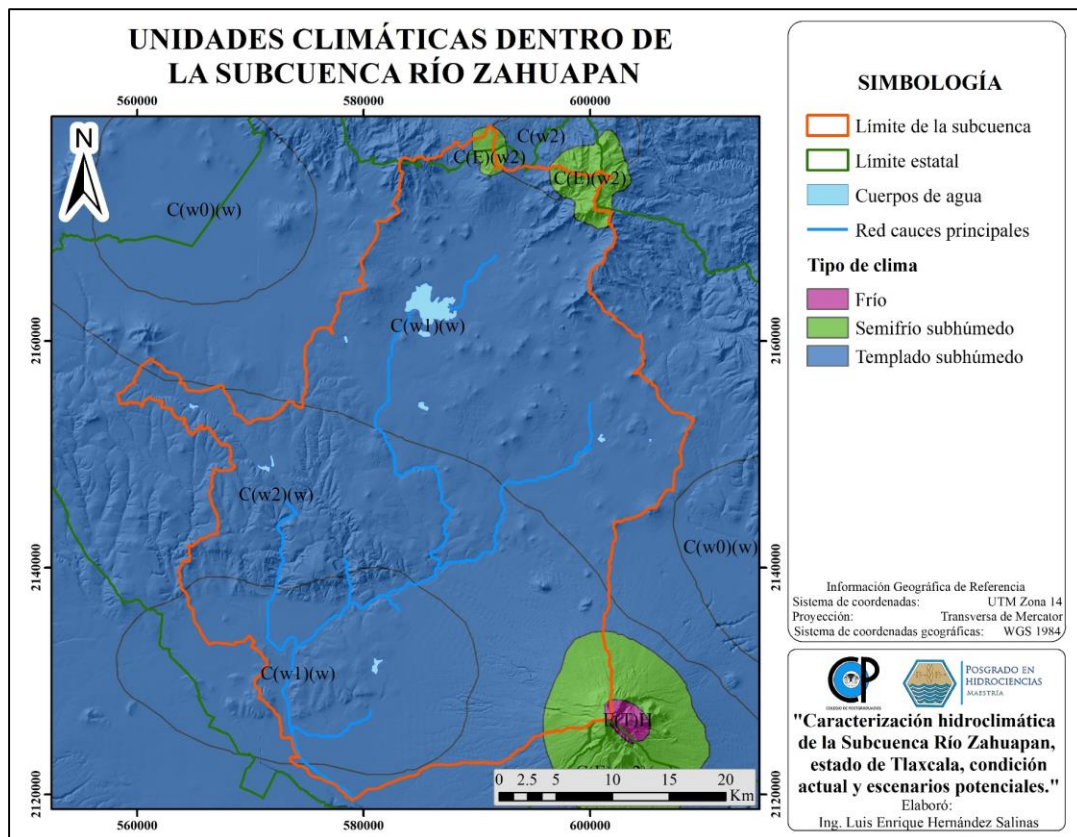
Figura 4.4.- Unidades Climáticas presentes en la subcuenca del río Zahuapan.
