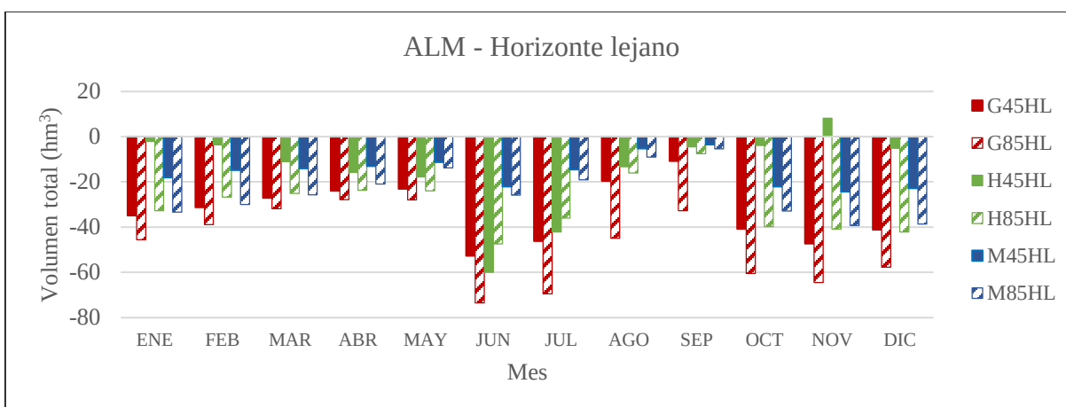
Figura 5.29.- Diferencia del volumen de agua almacenada en el suelo total en la subcuenca para los escenarios en el horizonte lejano (2075-2099) con respecto a la línea base.
