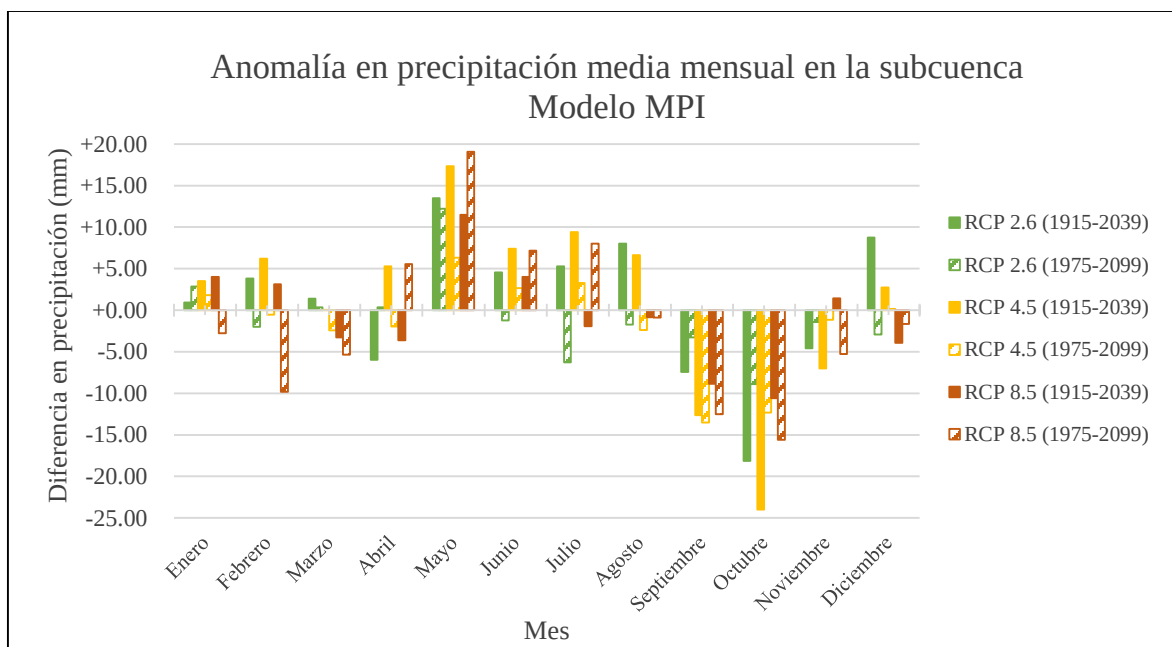
Figura 4.27.- Anomalía esperada en PP media mensual bajo MCG MPI_ESM_LR en la subcuenca.
