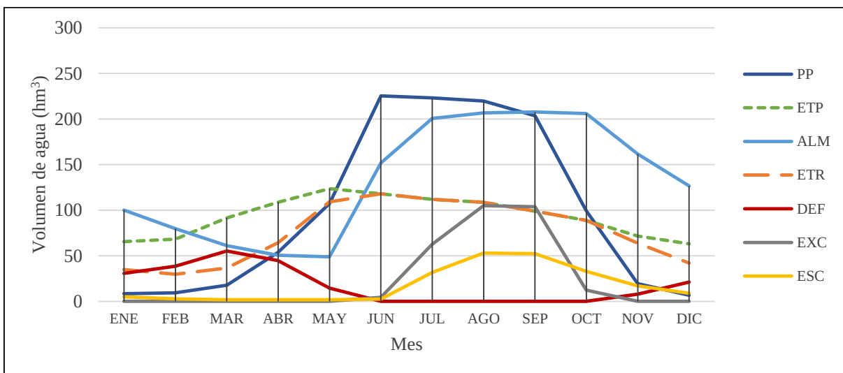
Figura 5.2.- Comportamiento del balance hídrico de la subcuenca río Zahuapan bajo el periodo de referencia 1984-2013.
