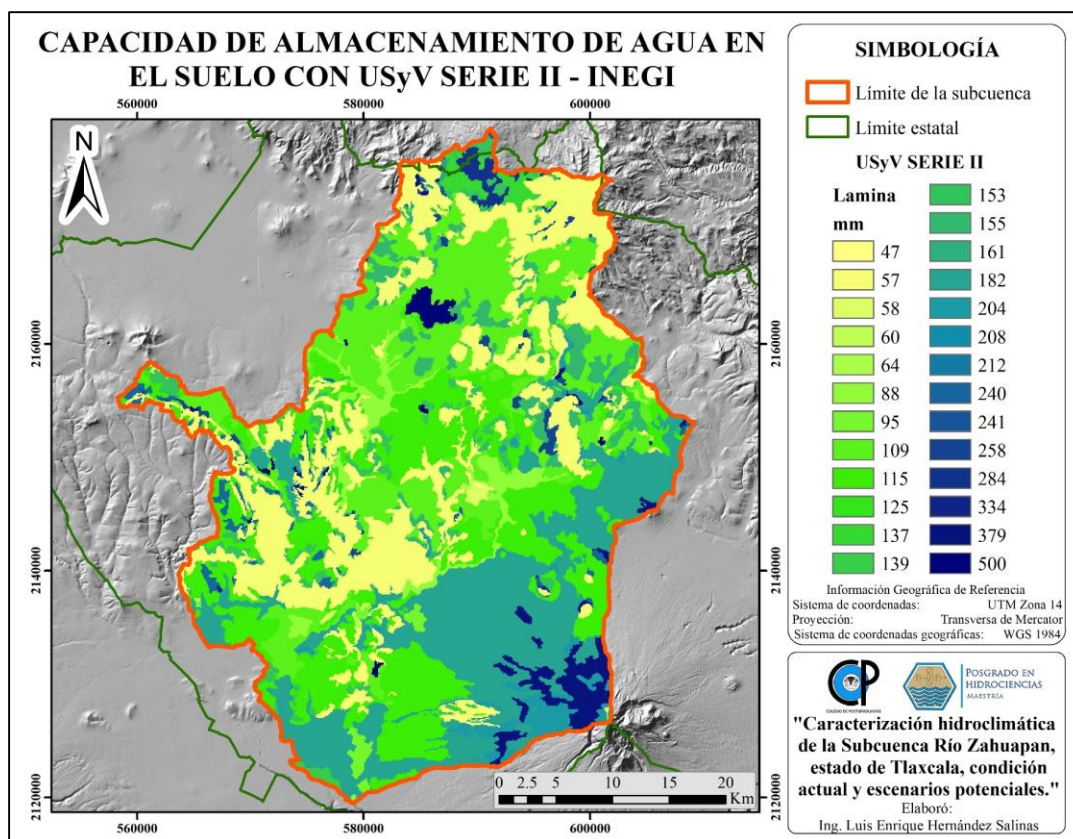
Figura 4.33.- Distribución final de la capacidad de almacenamiento de agua en el suelo; USyV Serie II - INEGI.
