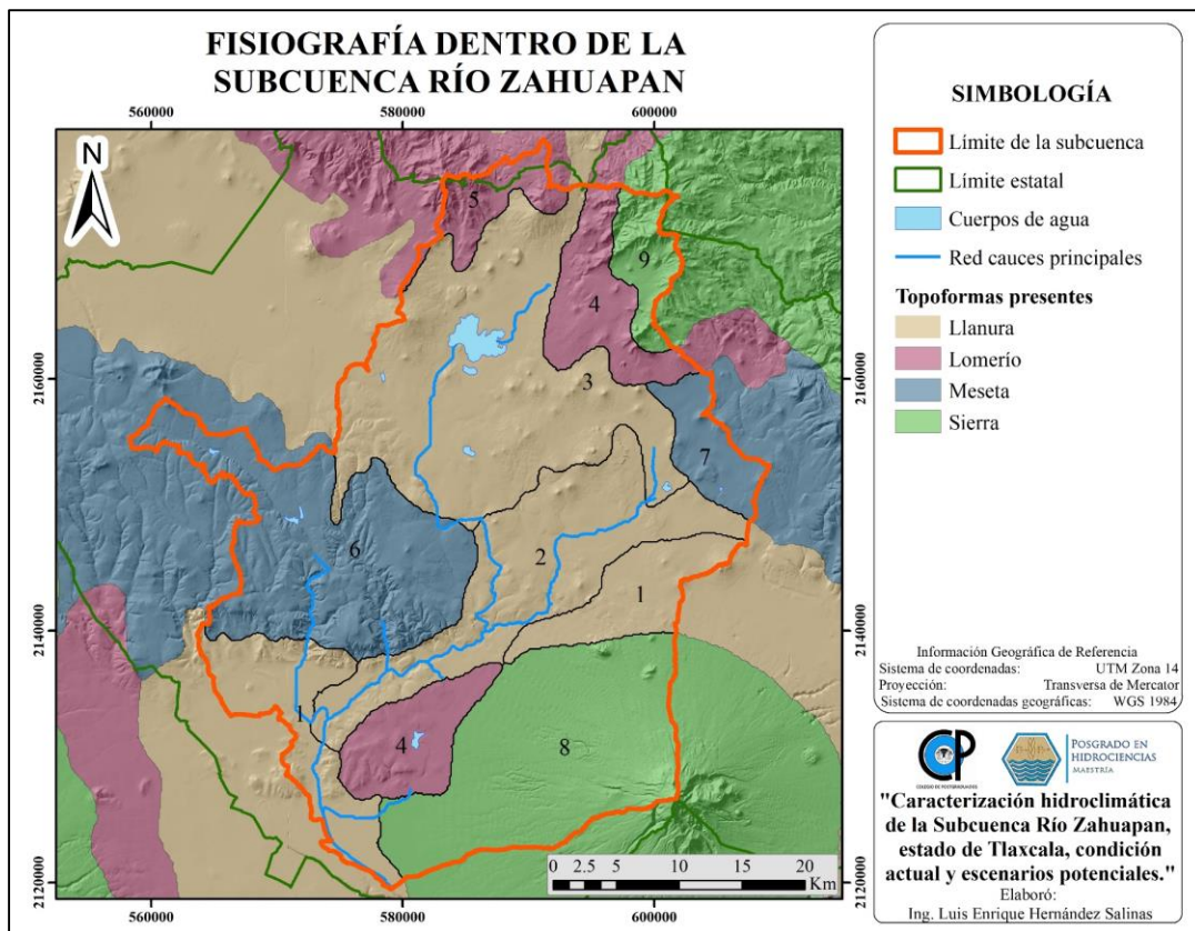
Figura 4.3.- Fisiografía de la subcuenca del río Zahuapan.
