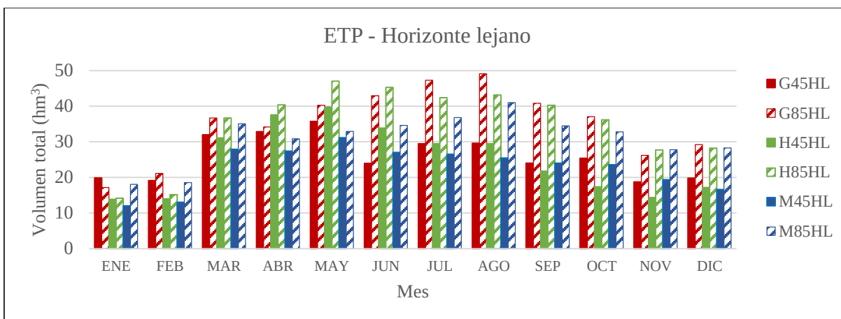
Figura 5.25.- Diferencia del volumen de evapotranspiración potencial total en la subcuenca para los escenarios en el horizonte lejano (2075-2099) con respecto a la línea base.
