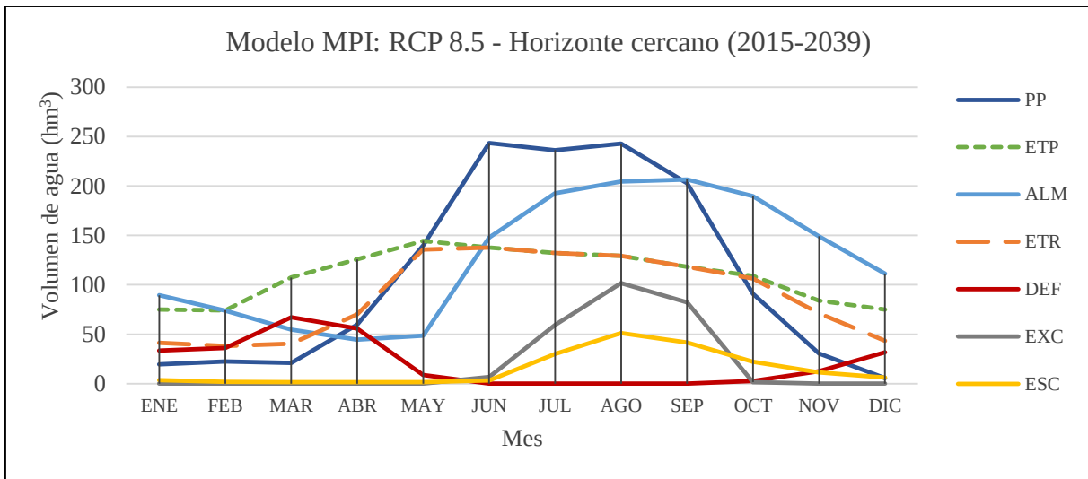
Figura 5.14.- Comportamiento del balance hídrico de la subcuenca río Zahuapan bajo el escenario RCP8.5 en el horizonte cercano (2015-2039) respectivo al modelo MPI.
