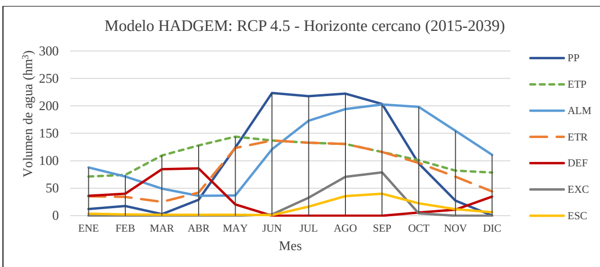
Figura 5.5.- Comportamiento del balance hídrico de la subcuenca río Zahuapan bajo el escenario RCP4.5 en el horizonte cercano (2015-2039) respectivo al modelo HADGEM.
