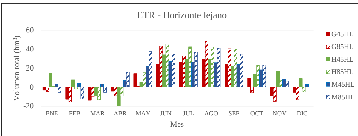
Figura 5.27.- Diferencia del volumen de evapotranspiración real total en la subcuenca para los escenarios en el horizonte lejano (2075-2099) con respecto a la línea base.
