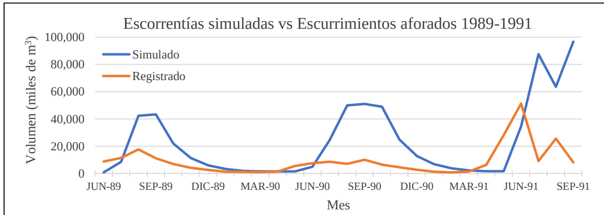
Figura 4.32.- Resultados de escorrentías simuladas contra escurrimientos aforados para la primera evaluación del código.
