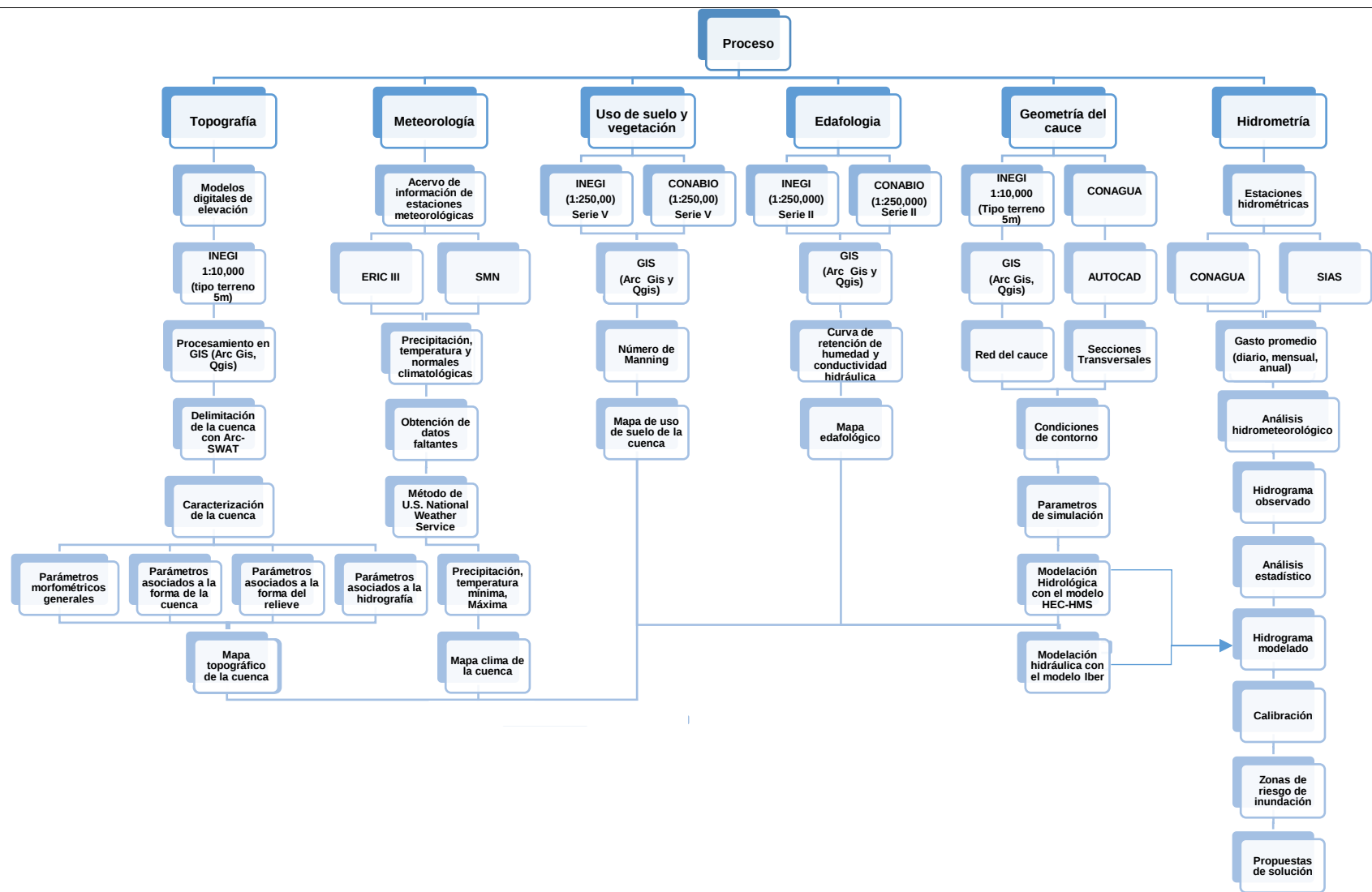
Figura 16. Metodología para la modelación con Iber
