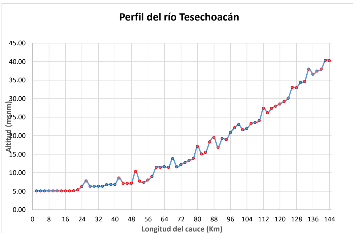
Figura 22. Perfil del cauce principal de la cuenca Tesechoacán
