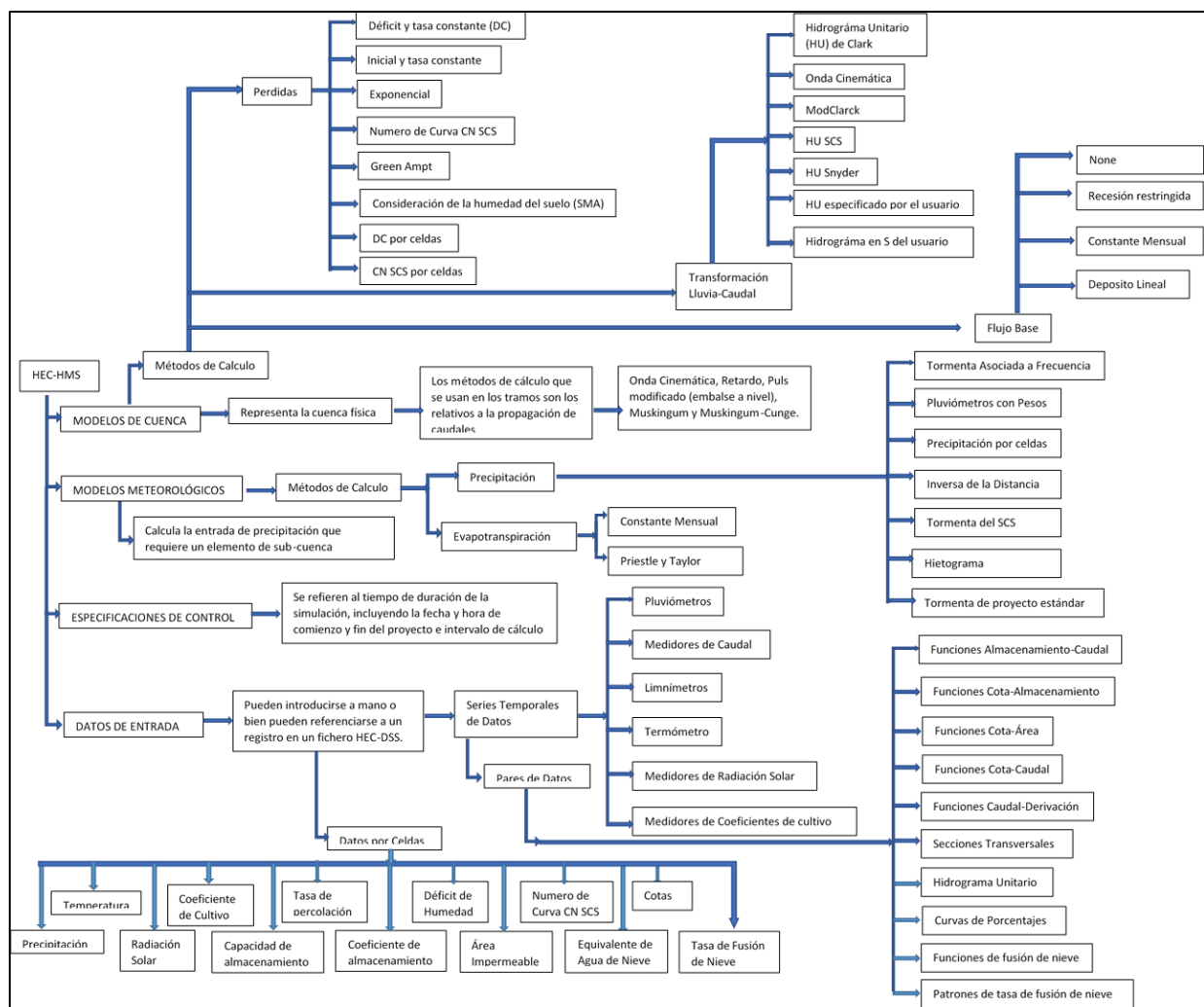
Figura 30. Diagrama teórico de HEC-HMS. Fuente: (Sánchez, 2016)
