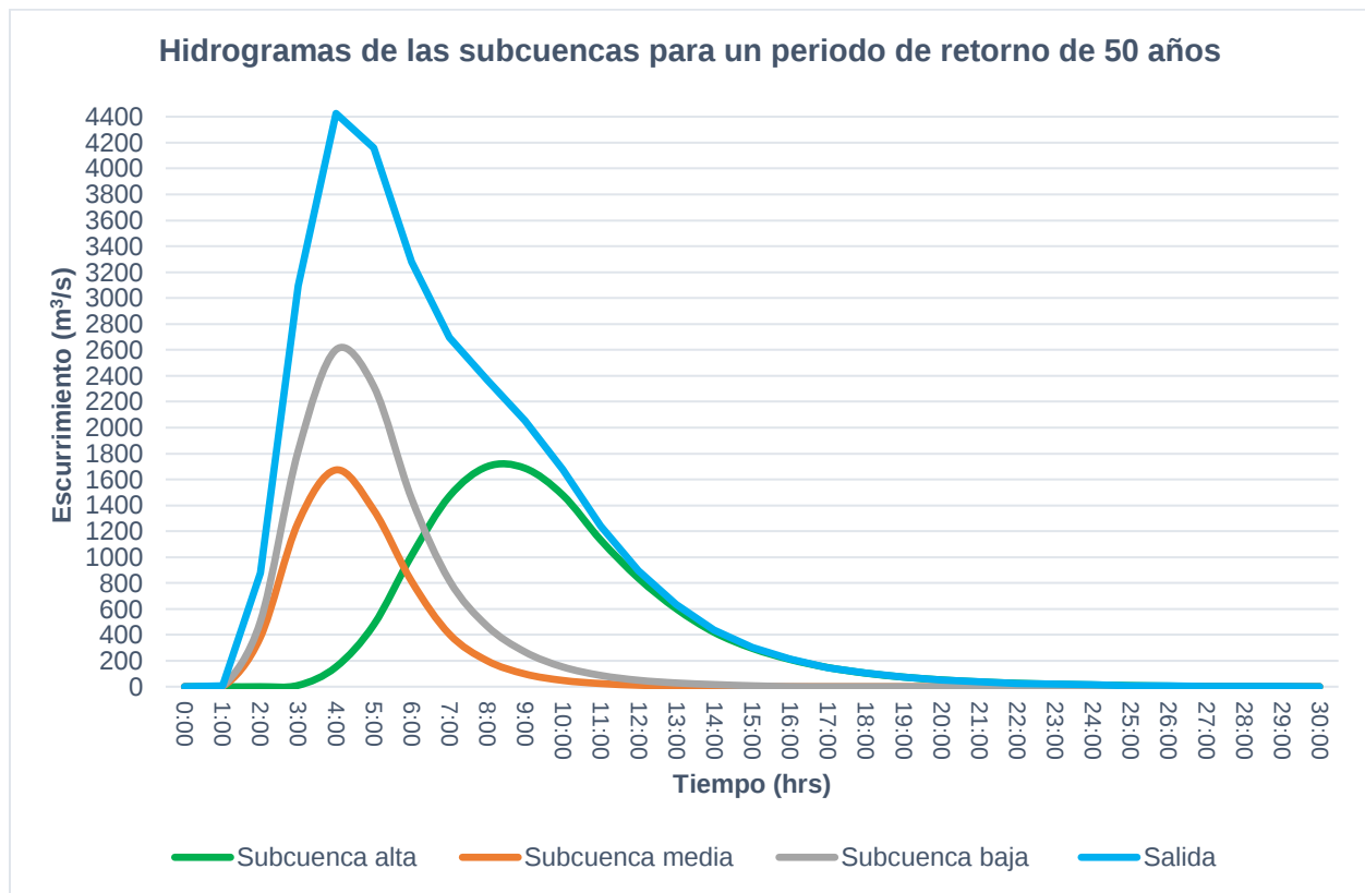
Figura 58. Hidrograma para un periodo de retorno de 50 años de la cuenca
