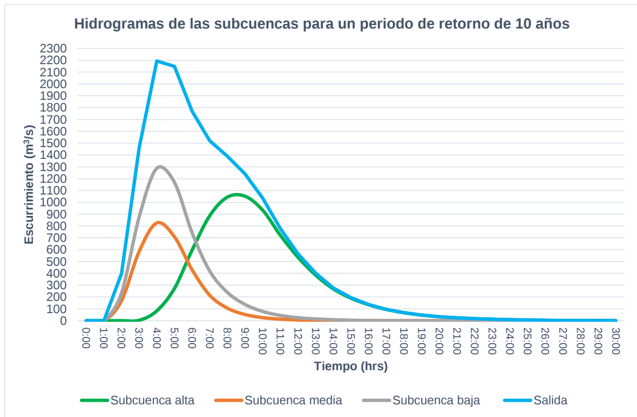
Figura 56. Hidrograma para un periodo de retorno de 10 años de la cuenca
