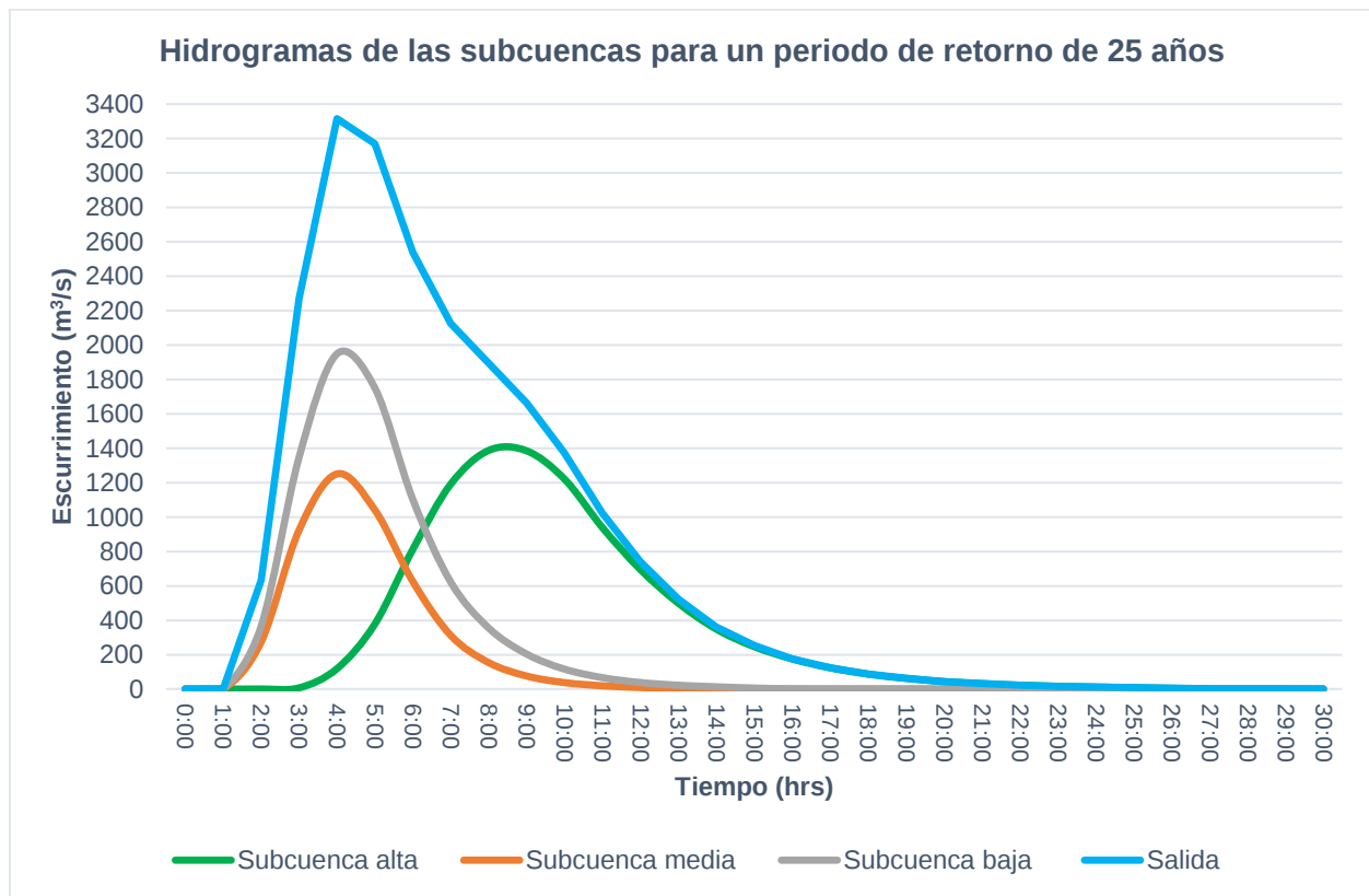
Figura 57. Hidrograma para un periodo de retorno de 25 años de la cuenca
