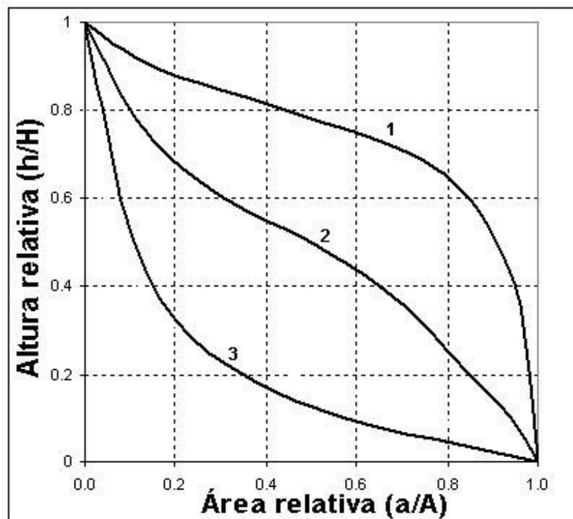
Figura 8. Curvas Hipsométricas. Fuente: (Campos, 1998)
