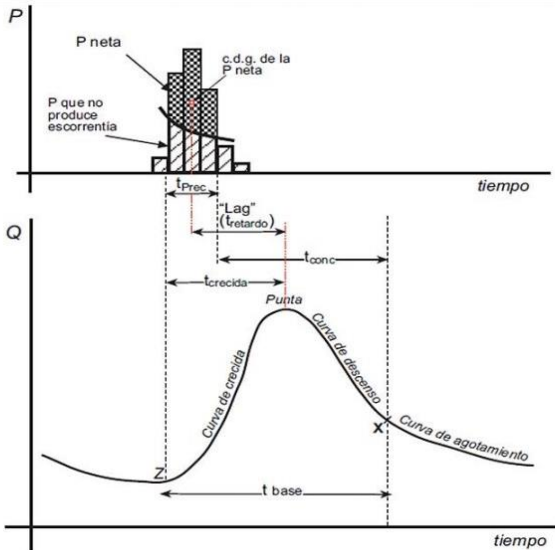
Figura 6. Partes de un hidrograma. Fuente: (Aparicio, 2005)
